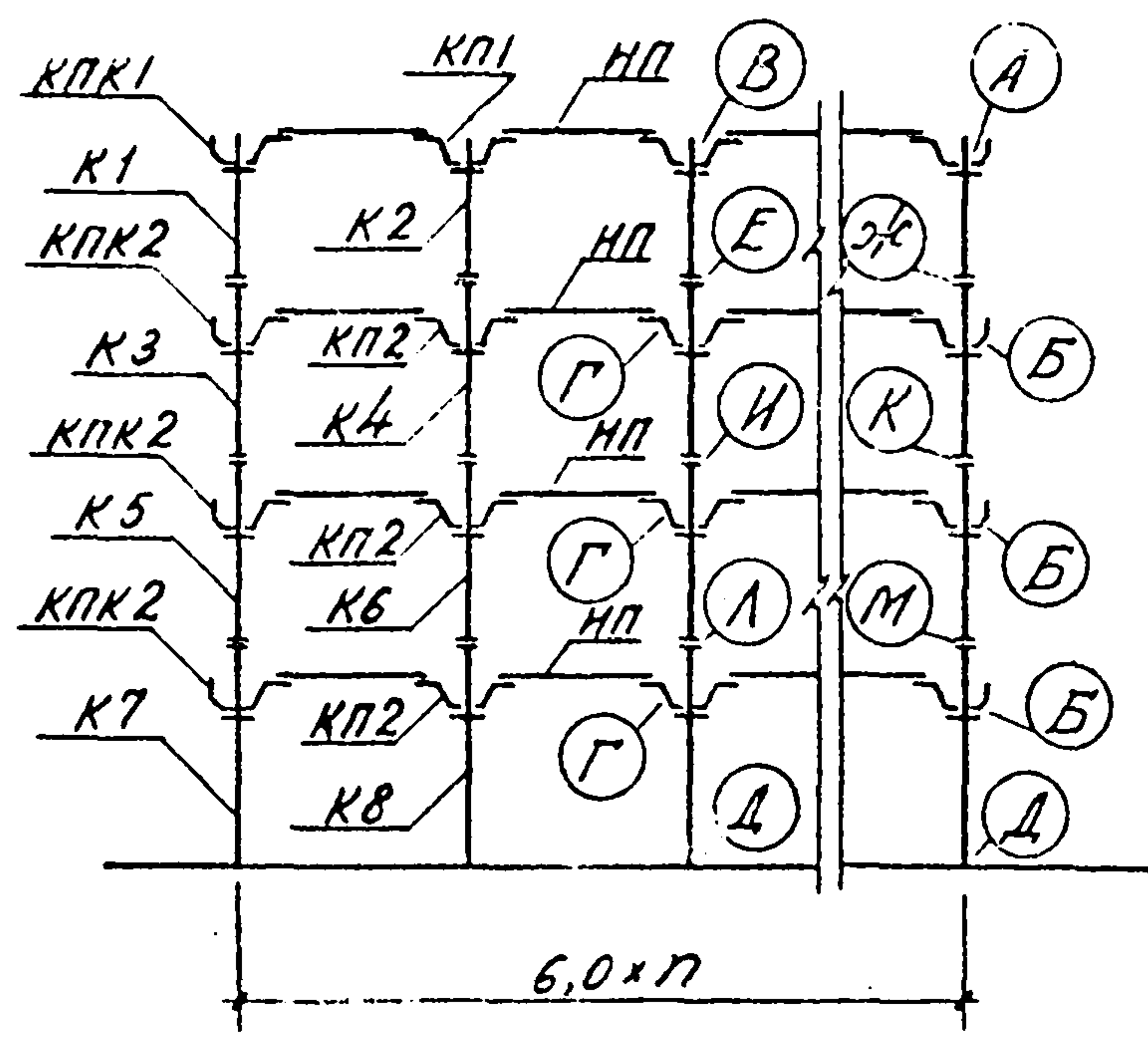
Схема рамы 6-06-n-4 (4,8)
