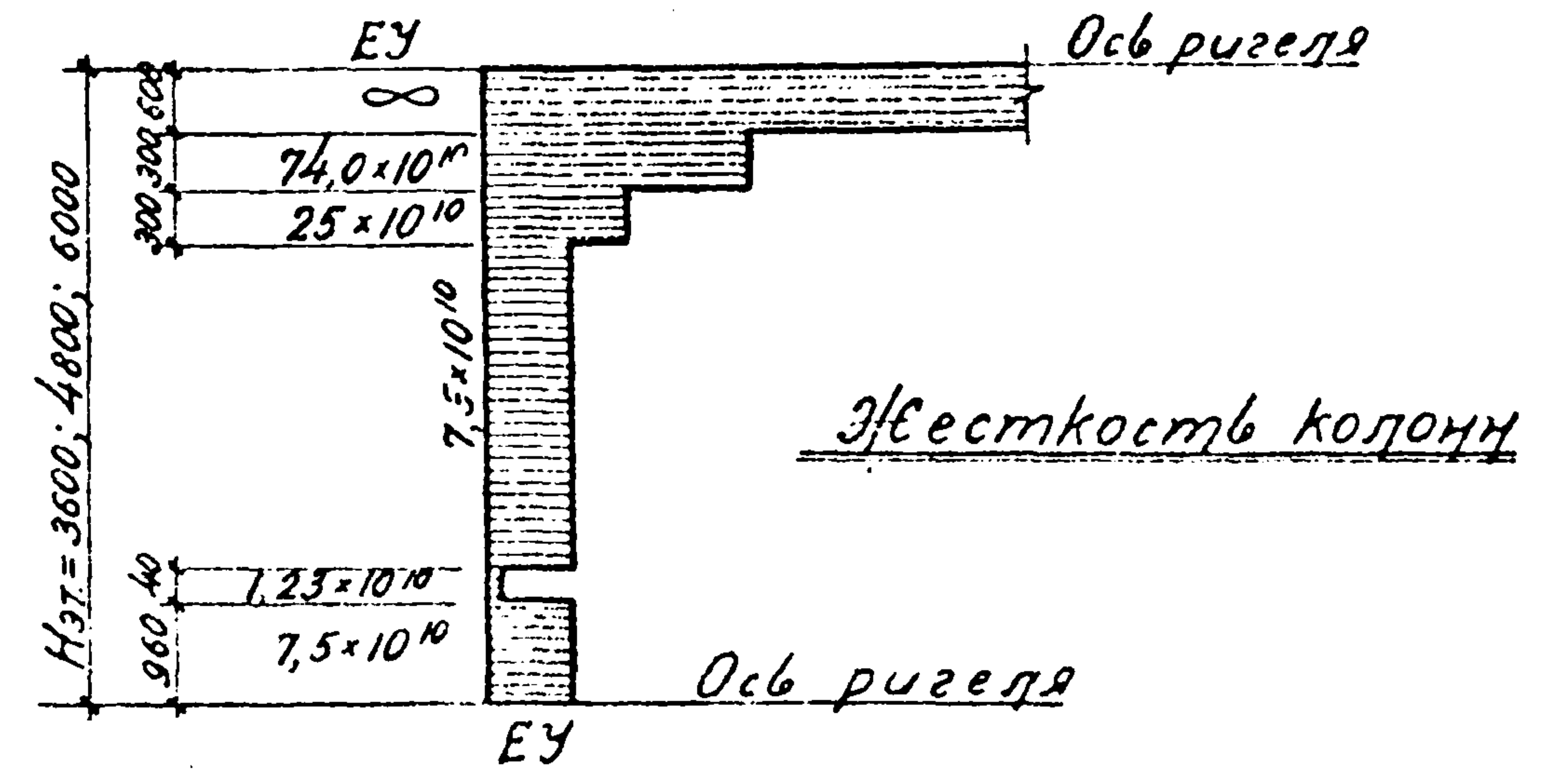
Жесткости конструкций на стадии монтажа (кгсм 2 ) Чертеж №2
