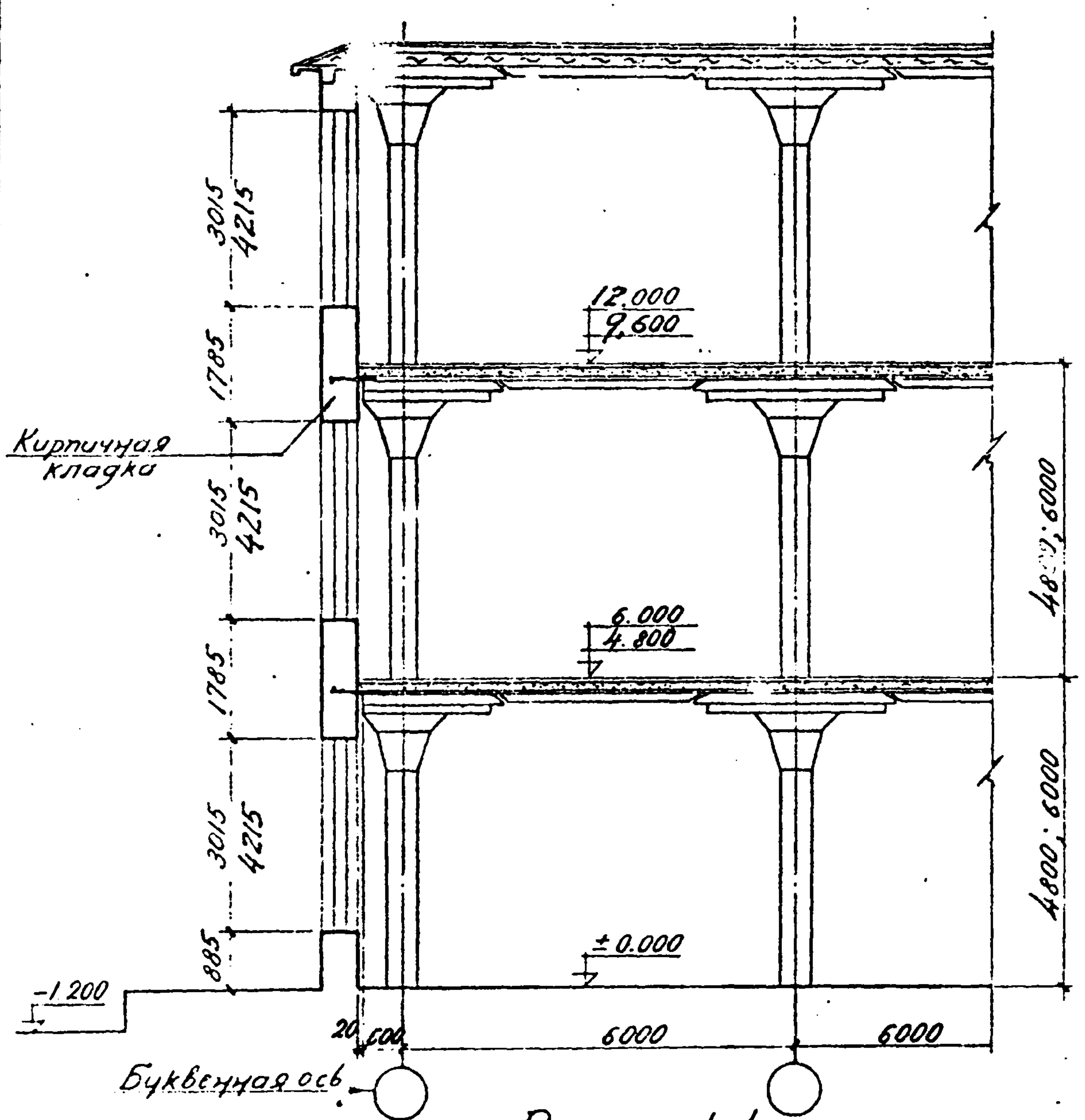
Разрез 1-1
