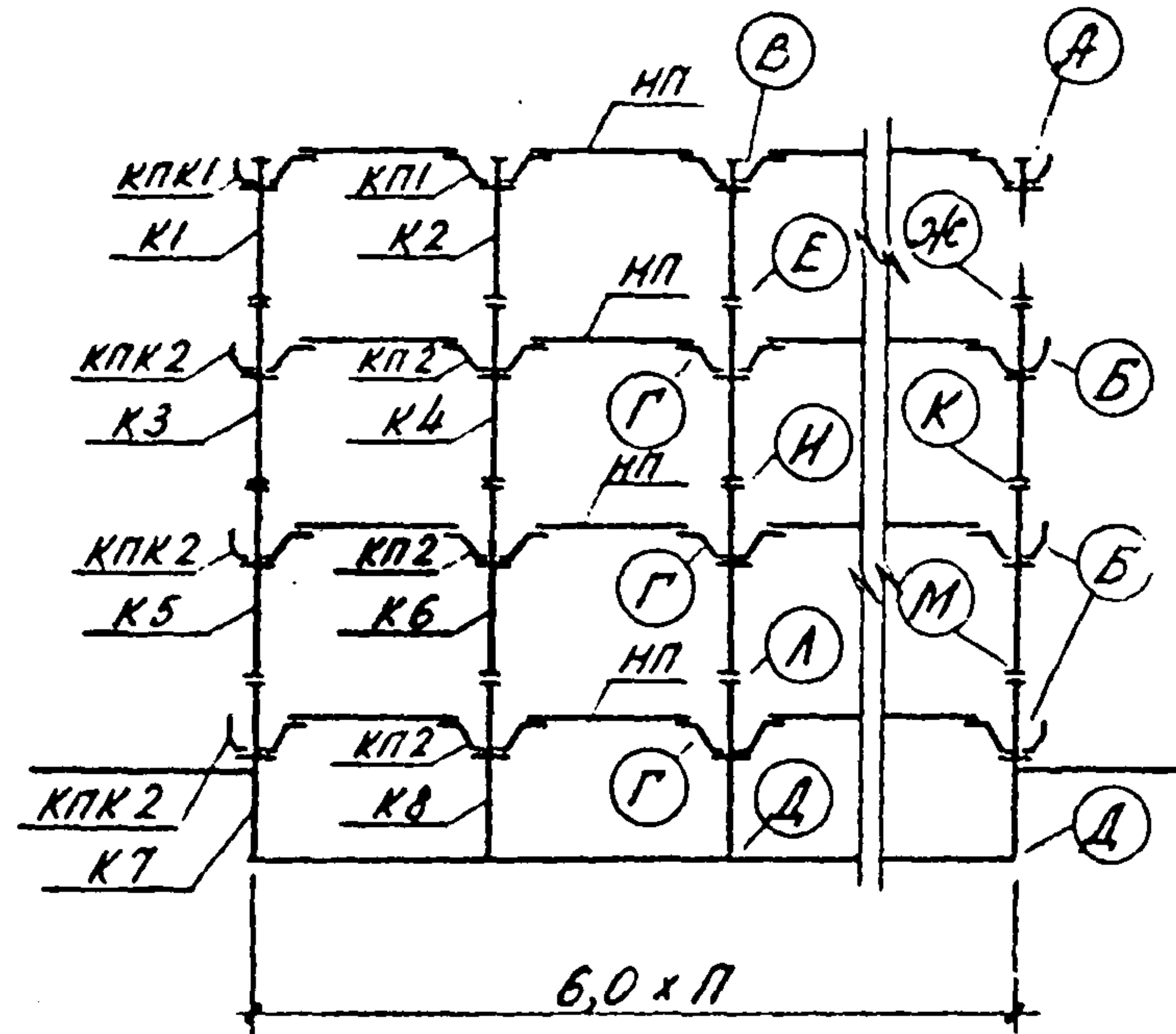
Схема рамы 6-0,6-п-3+подвал (4,8; 4,8; 3,6)
