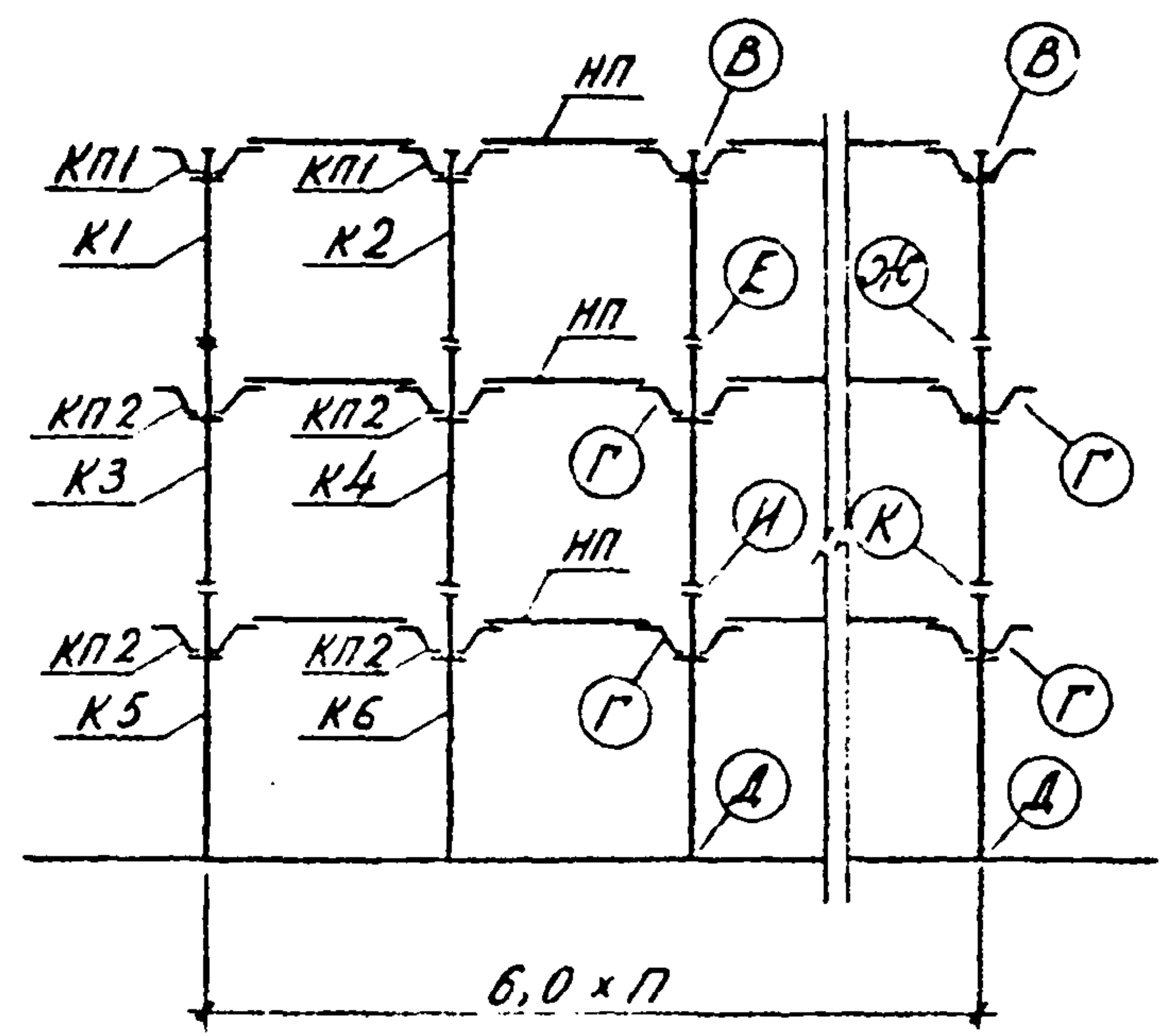
Схема рамы 6-1,55-П-3 (6,0)
