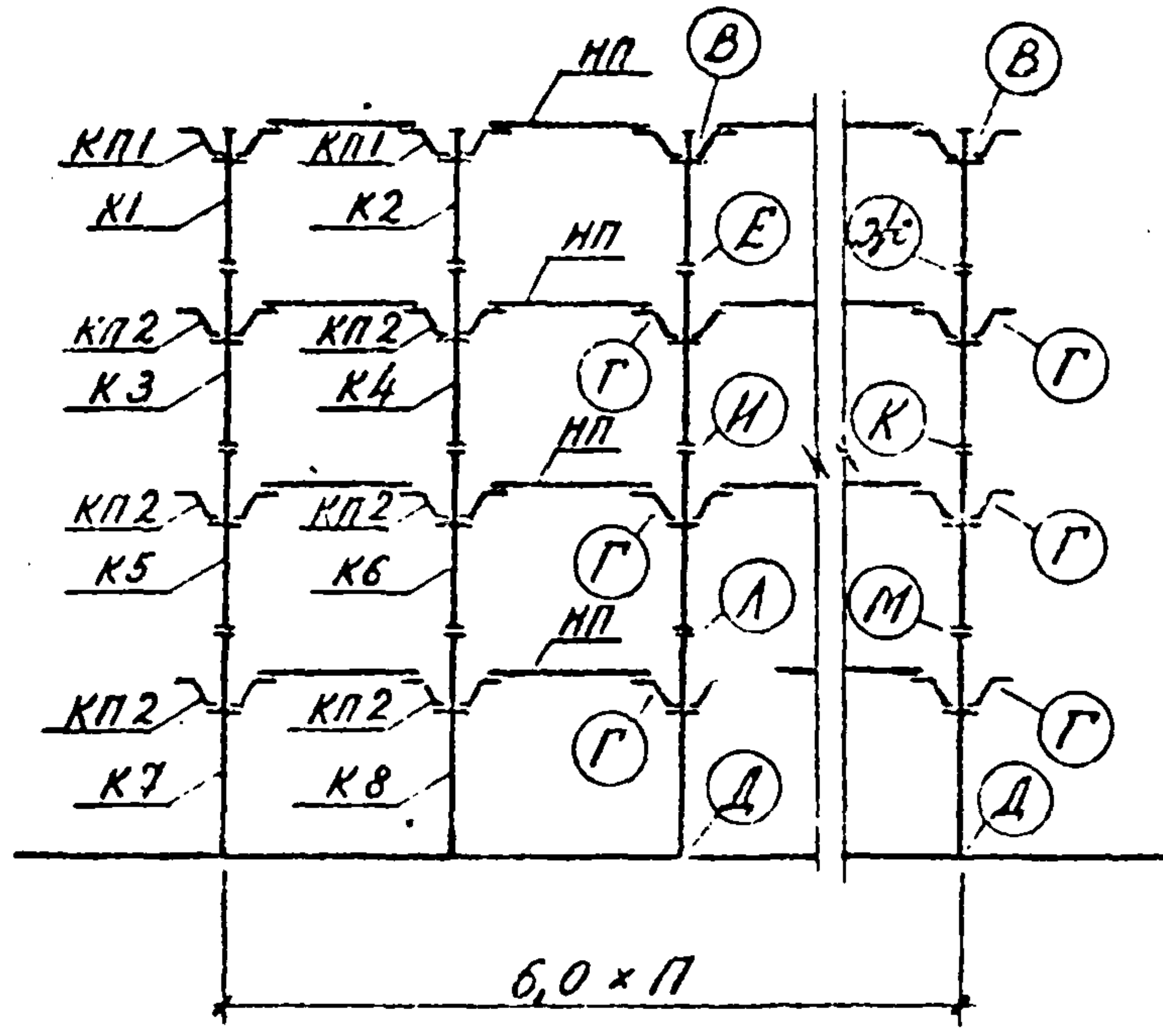
Схема рамы 6-1,55-П-4 (4,8)
