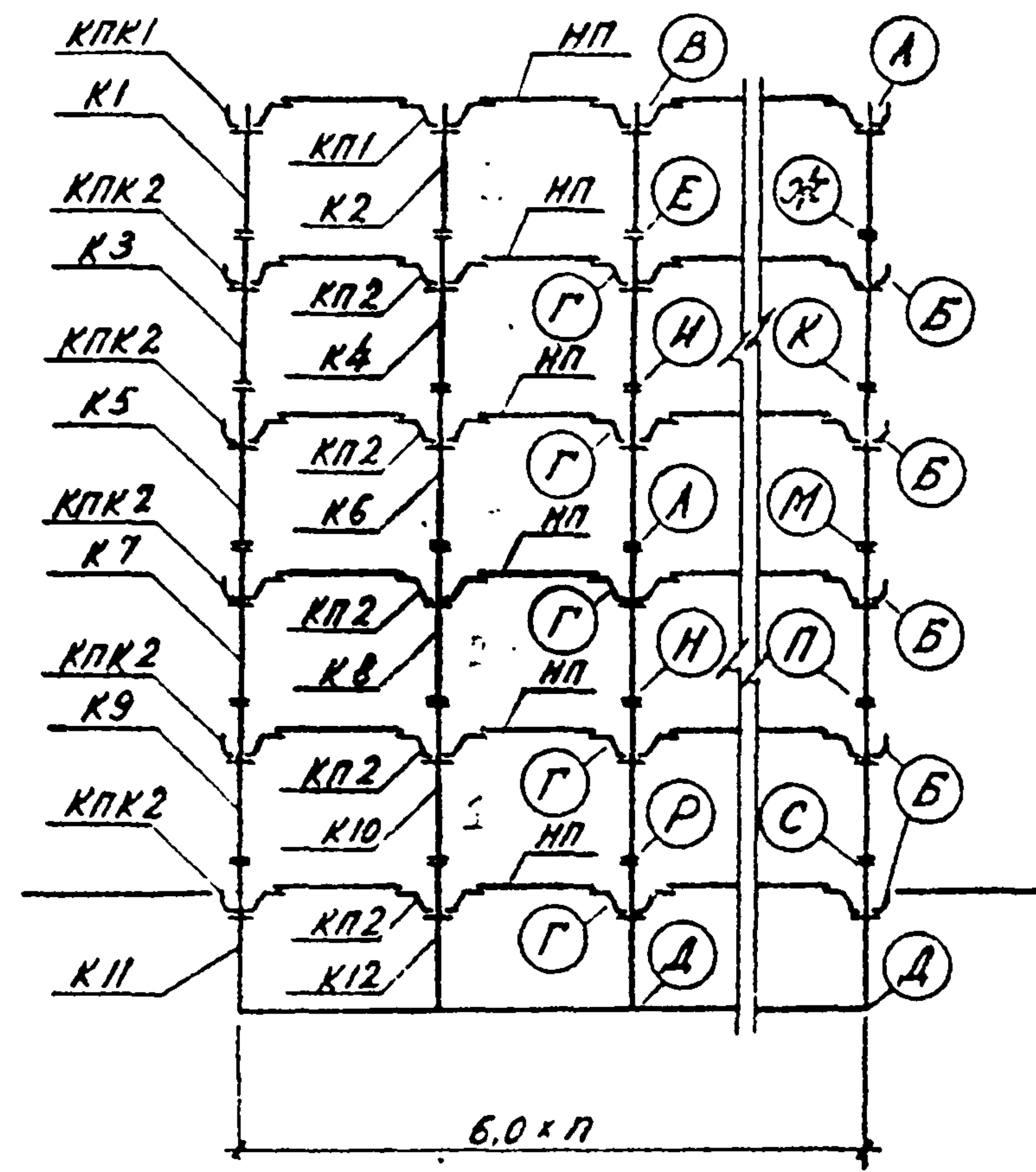
Схема рамы 6-0,6-n-5+подвал (4,8; 4,8; 3,6)
