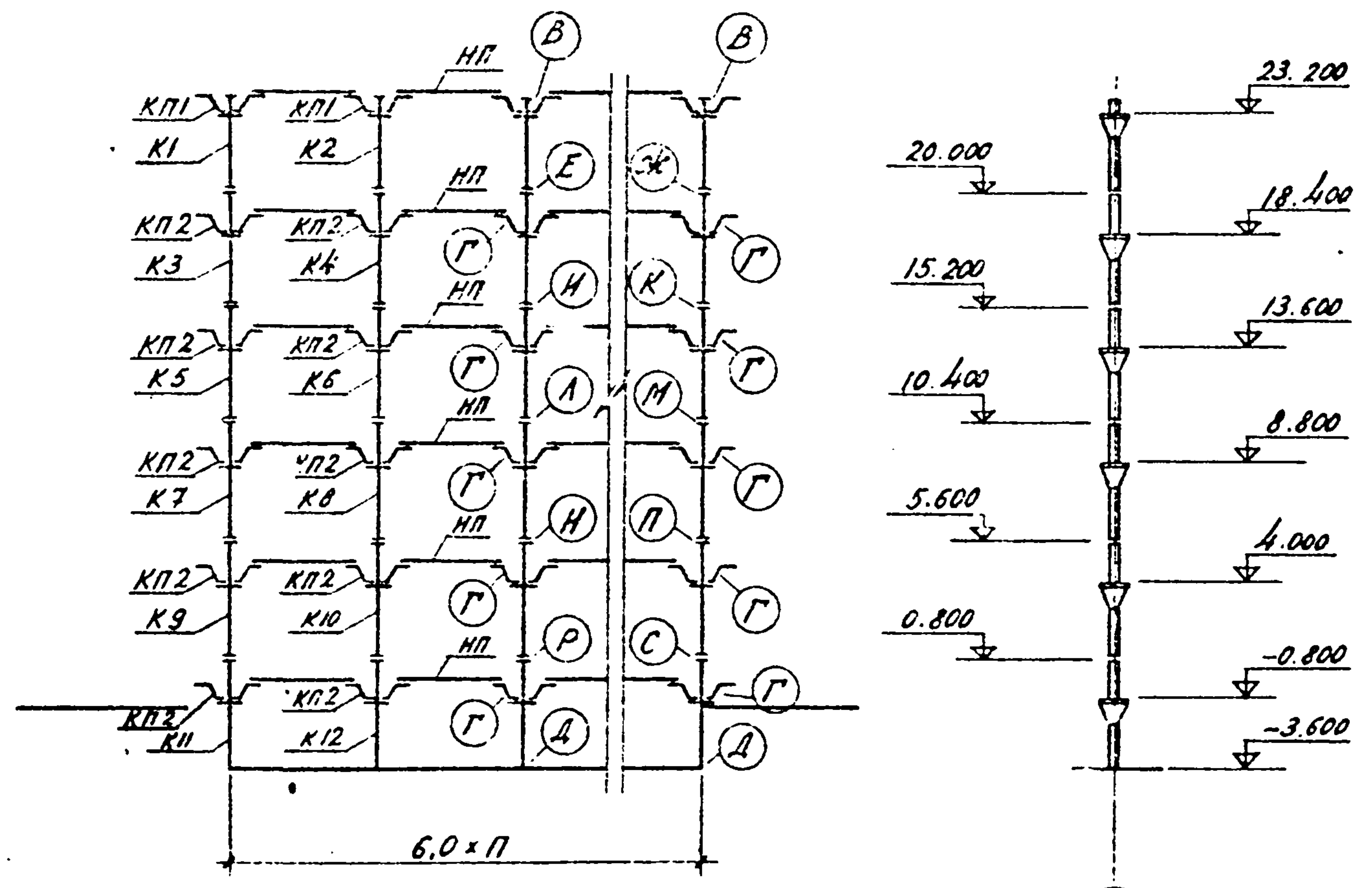
Схема рамы 6-1,55-П-5+подвал (4,8;4,8;3,6)
