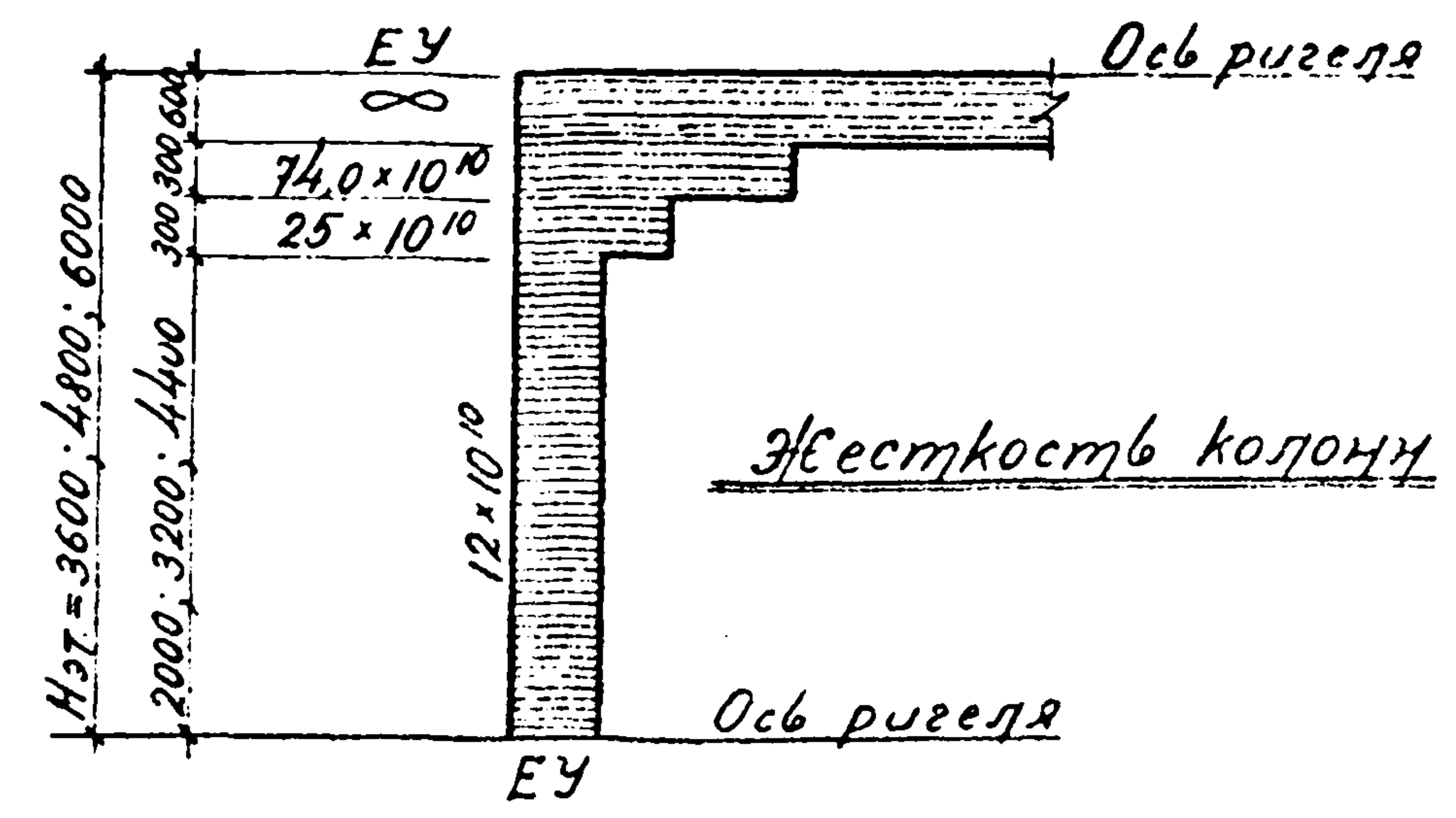
Жесткости конструкций в эксплуатационной стадии (кгсм 2 ) Чертеж №1
