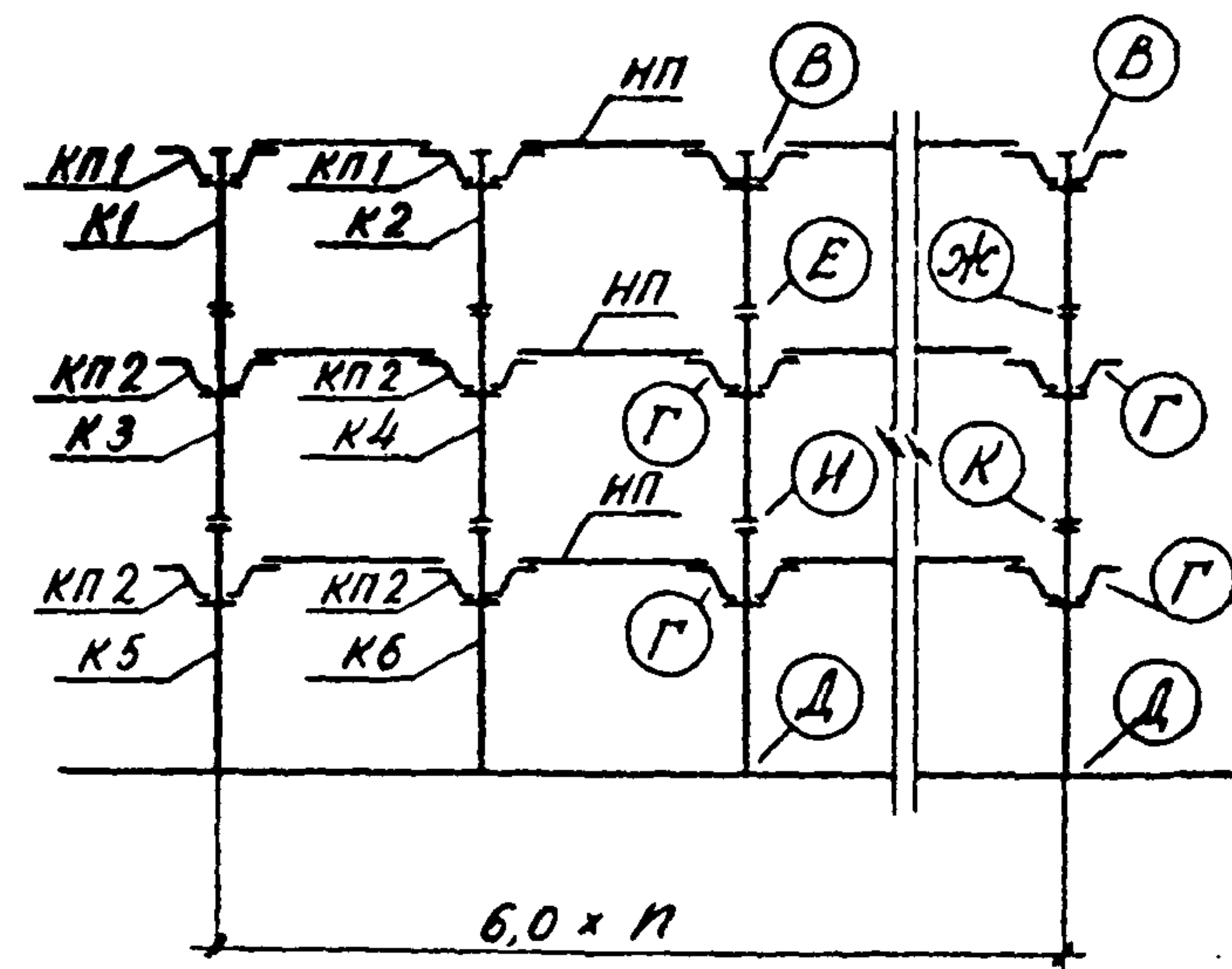
Схема рамы 6-1,55-п-3 (4, 8)
