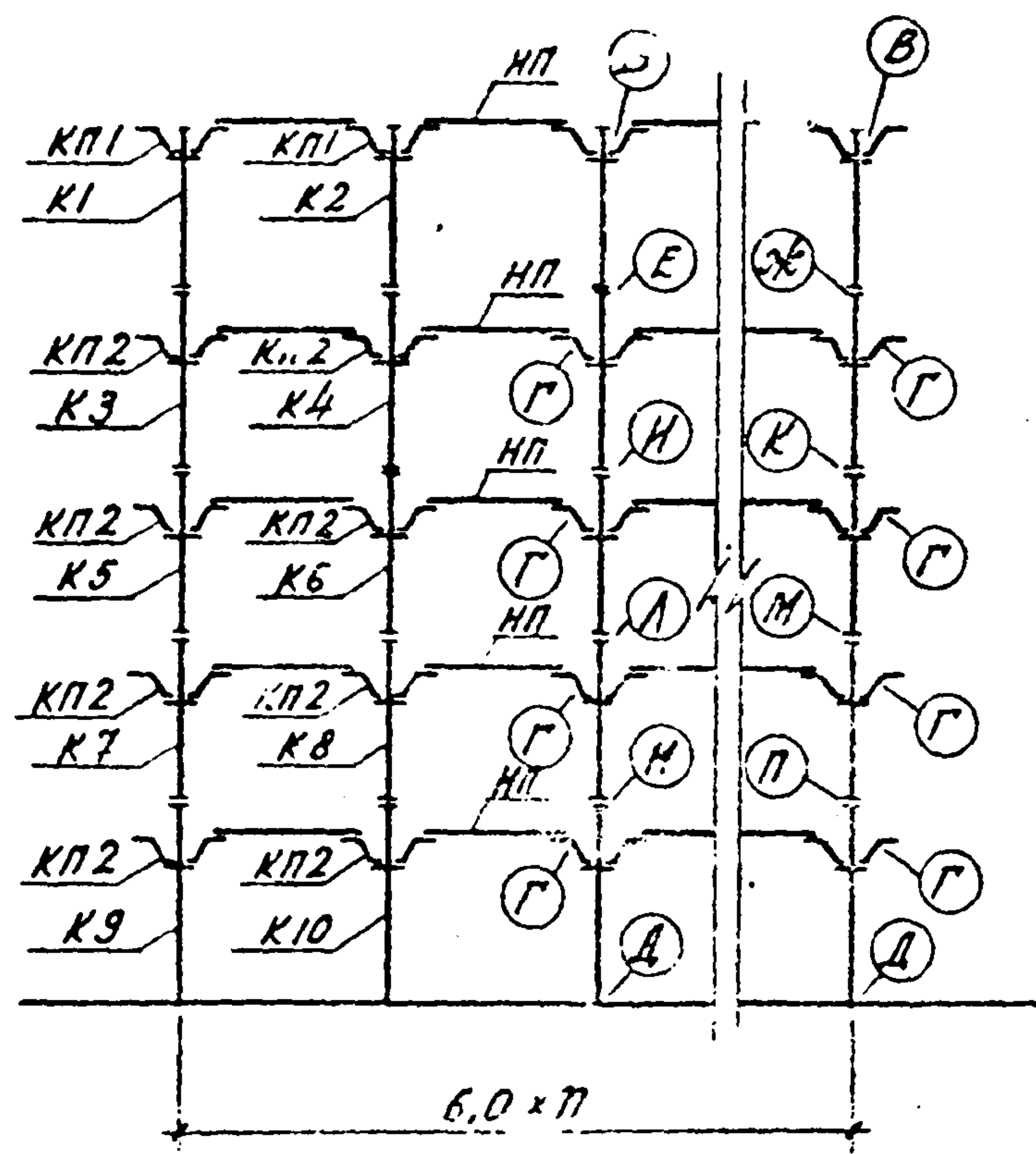
Схема рамы 6-1,55-П-5 (6,0; 4,8; 4,8)
