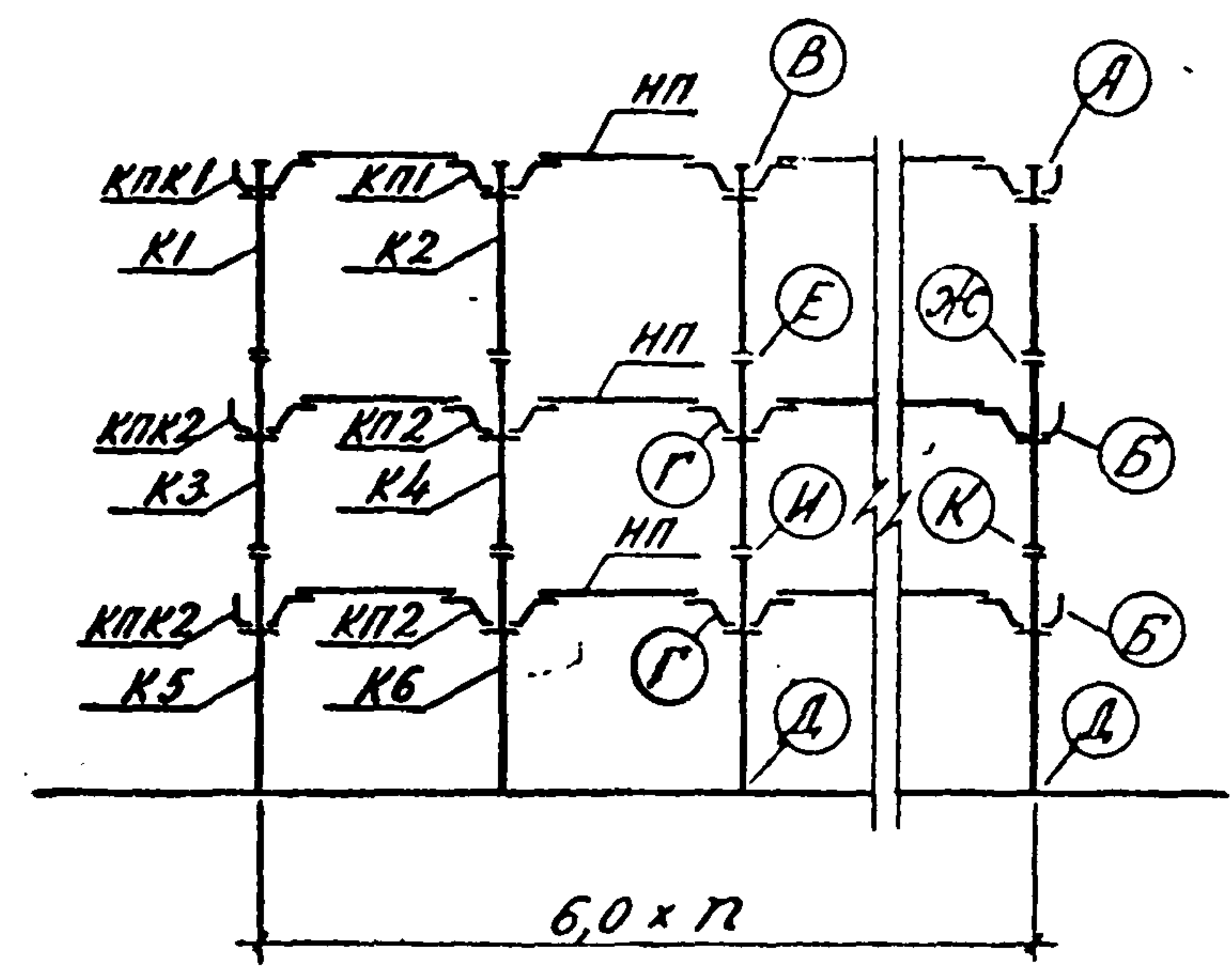
Схема рамы 6-0,6-п-3 (6,0; 4,8; 4,8)
