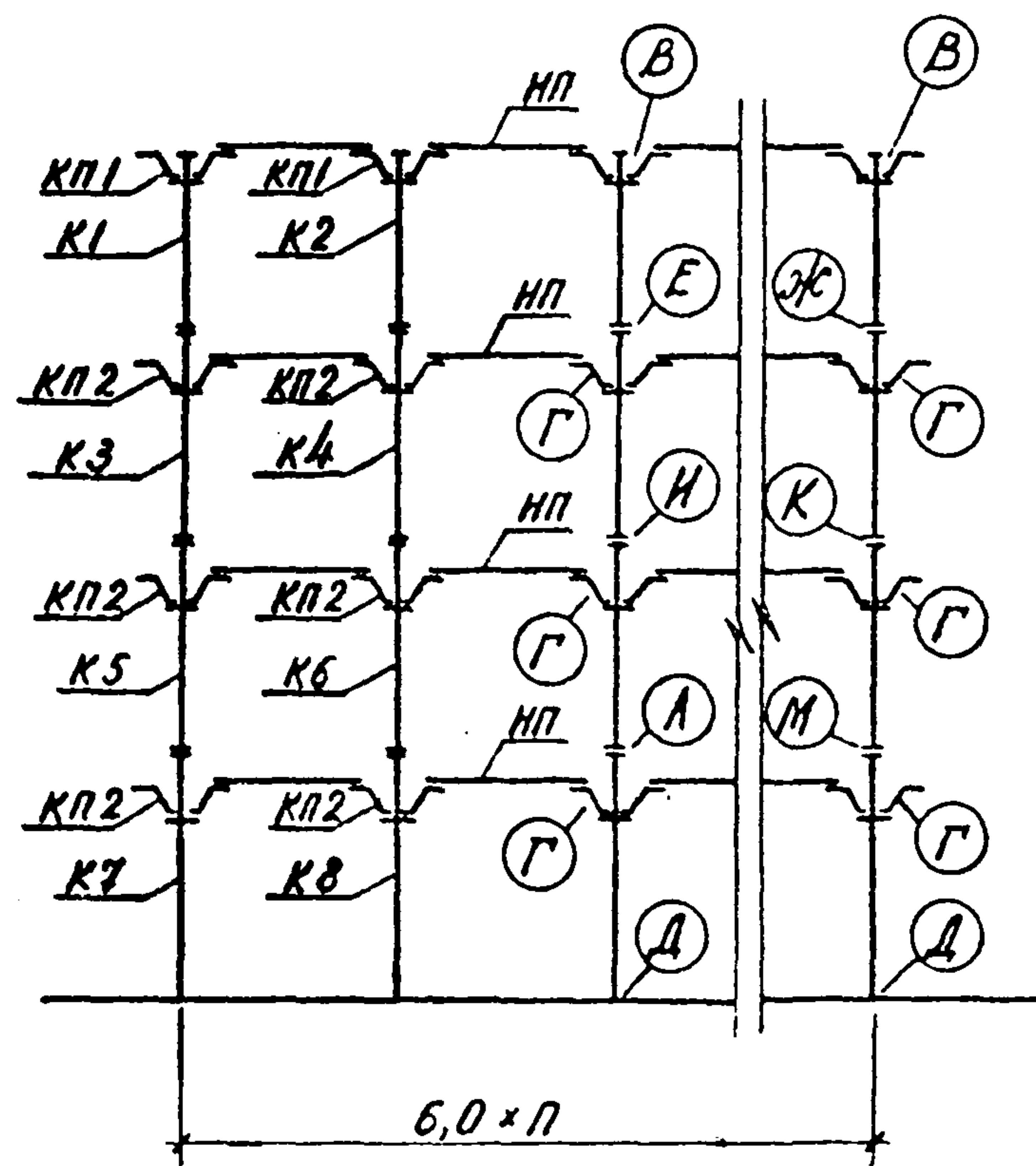
Схема рамы 6-1,55-п-4 (6,0)
