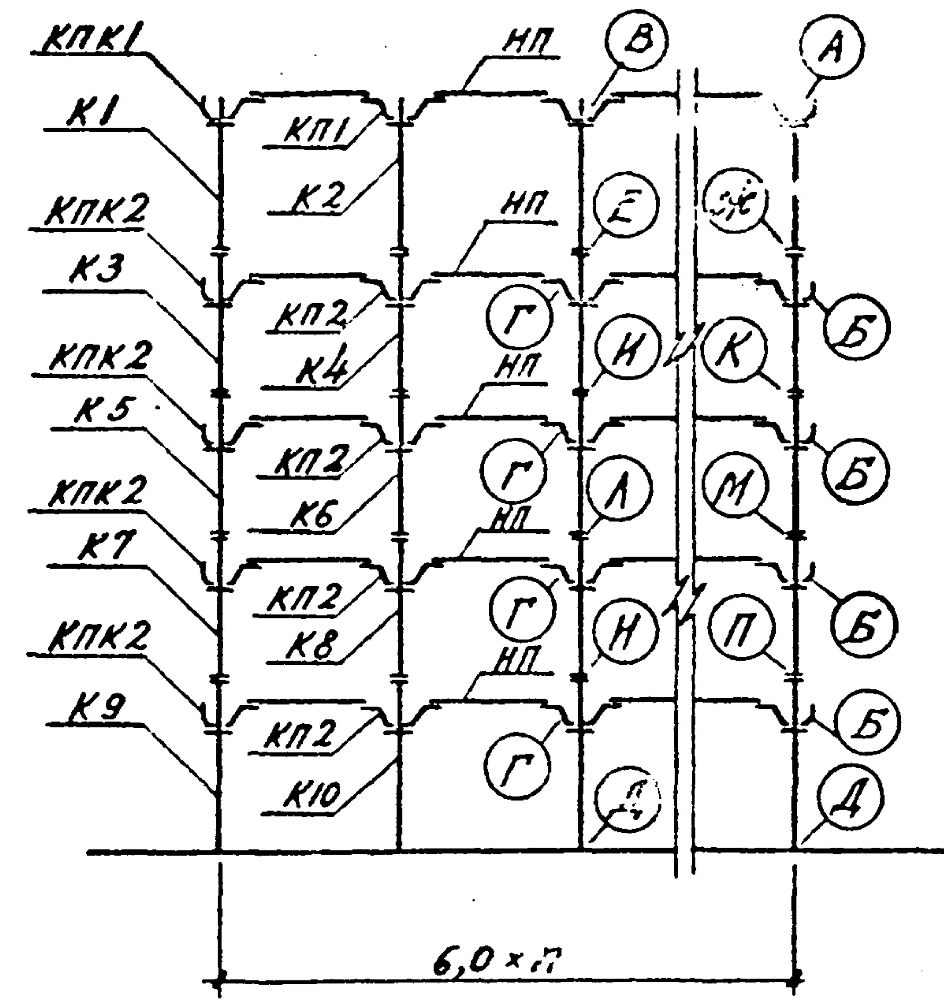
Схема рамы 6-0,6-П-5(6,0; 4,8; 4,8)
