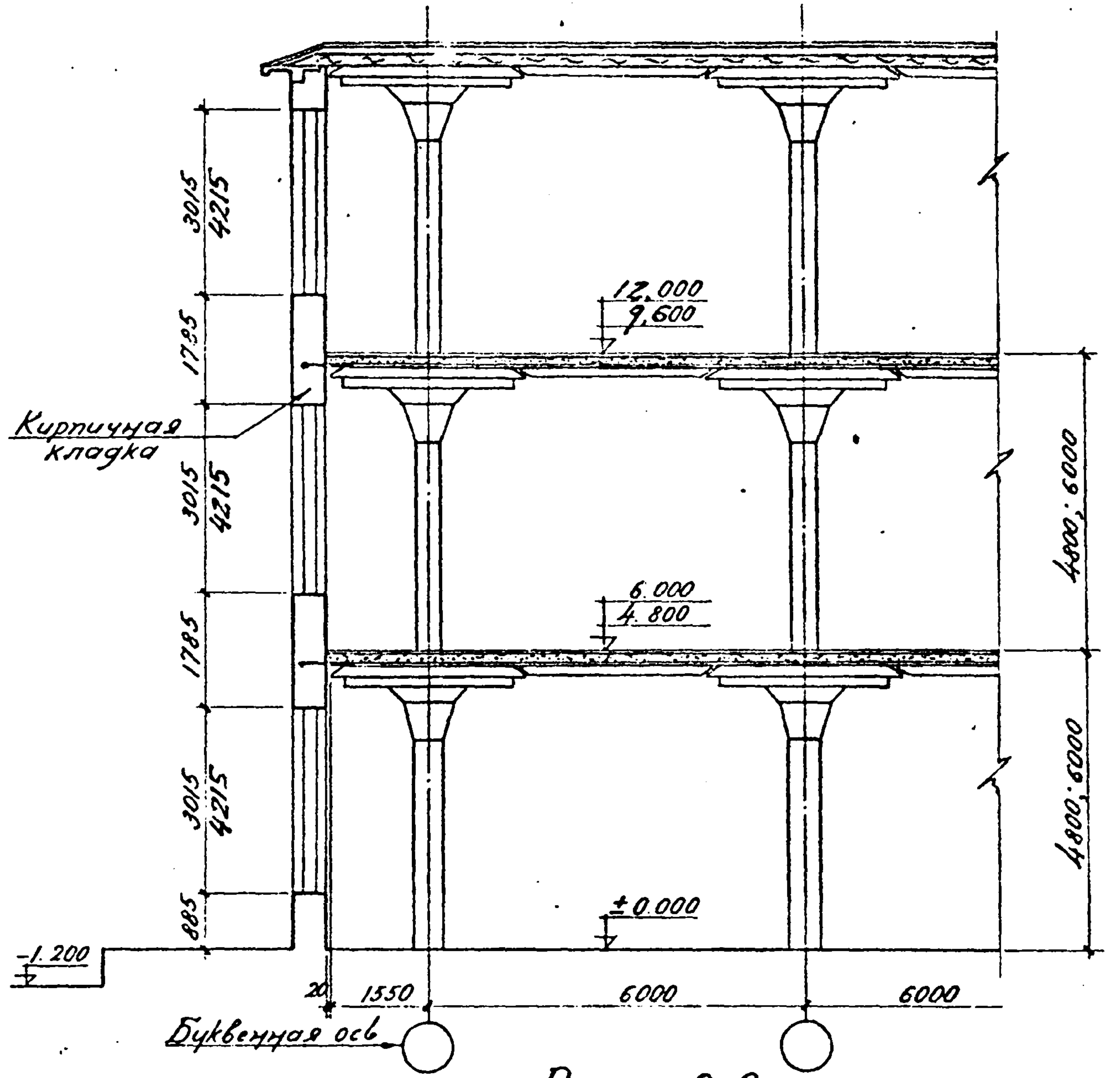
Разрез 2-2
