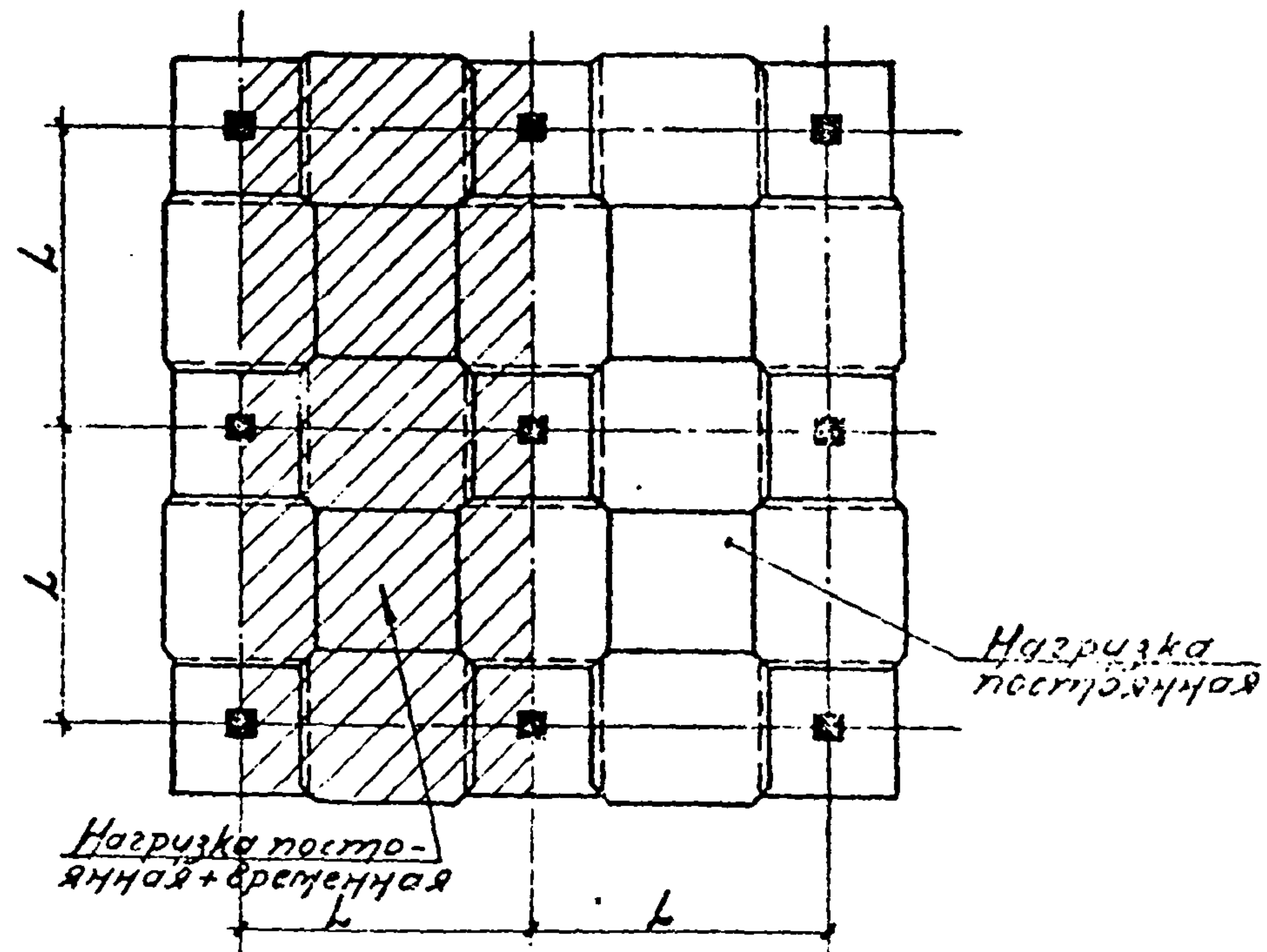
Чертеж №3
