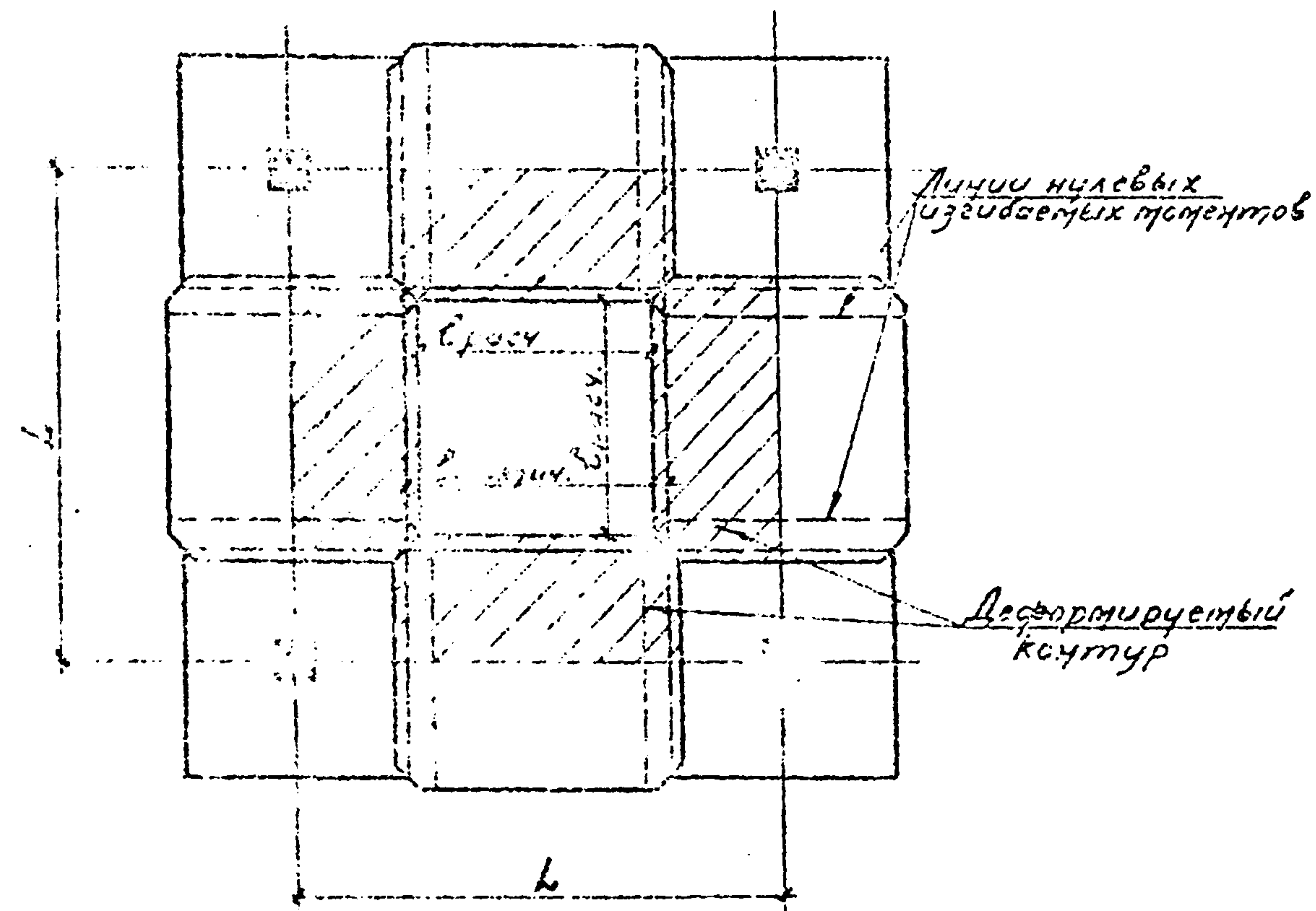
Чертеж №6
