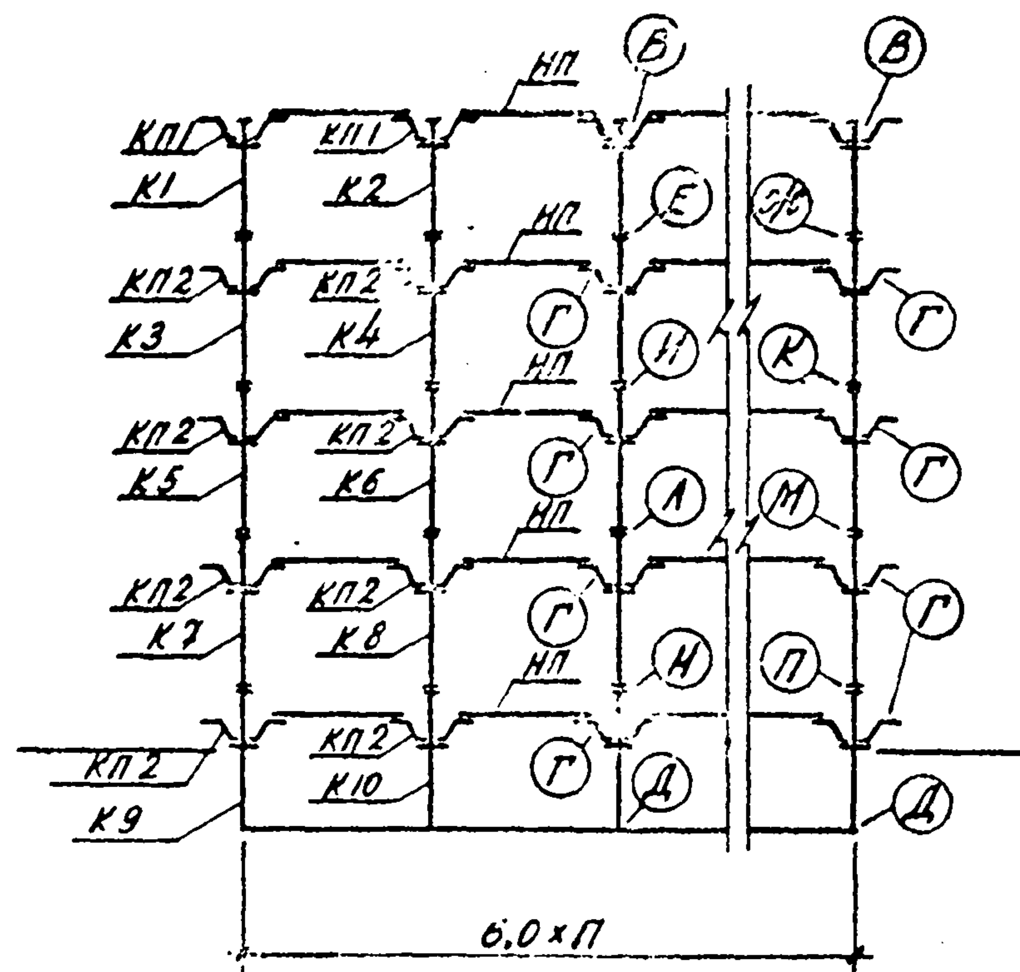
Схемы рамы 6-1.55-П-4+подвал(4,8;4,8;3,6)
