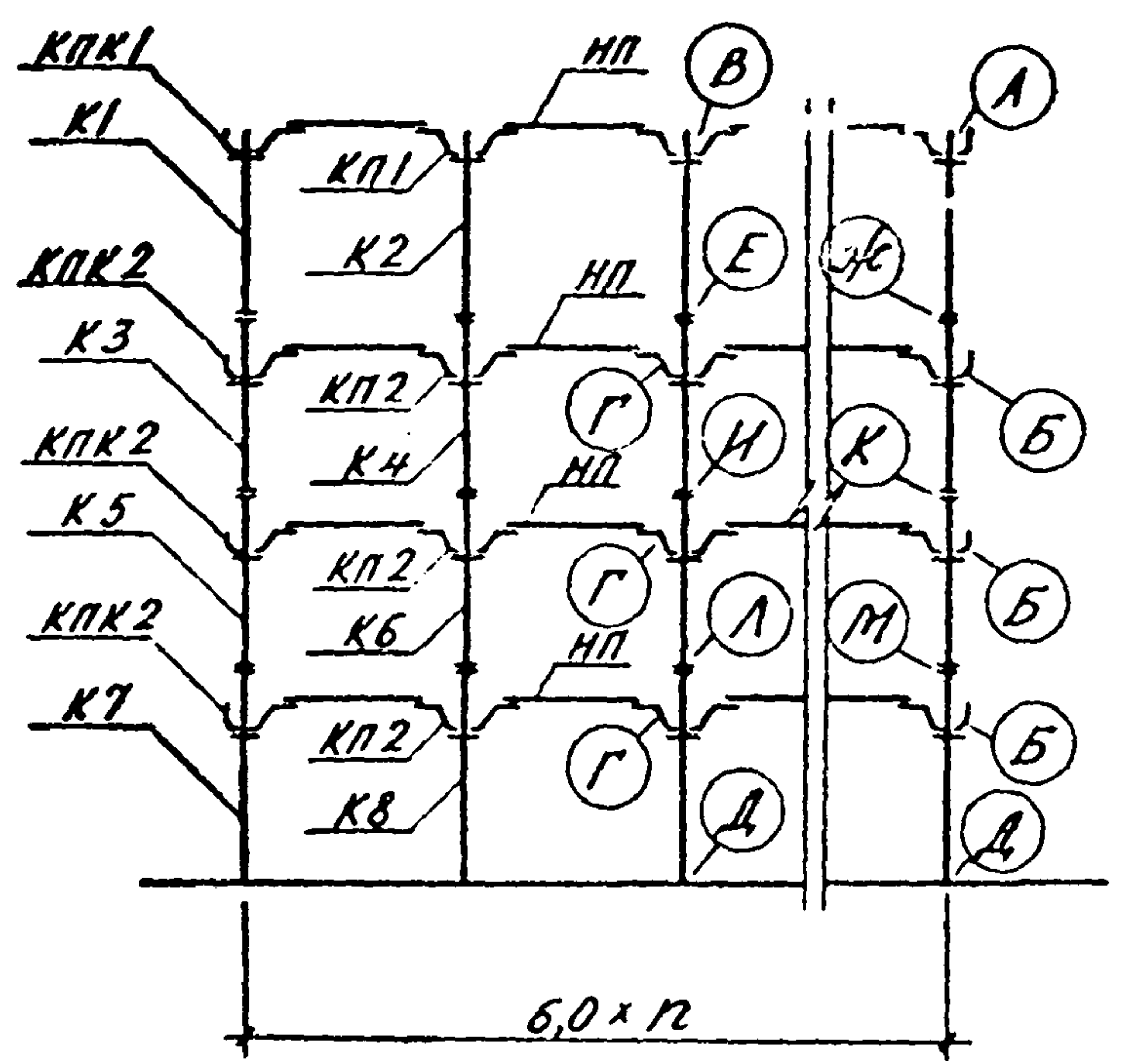
Схема рамы 6-06-п-4(6,0;4,8;4,8)
