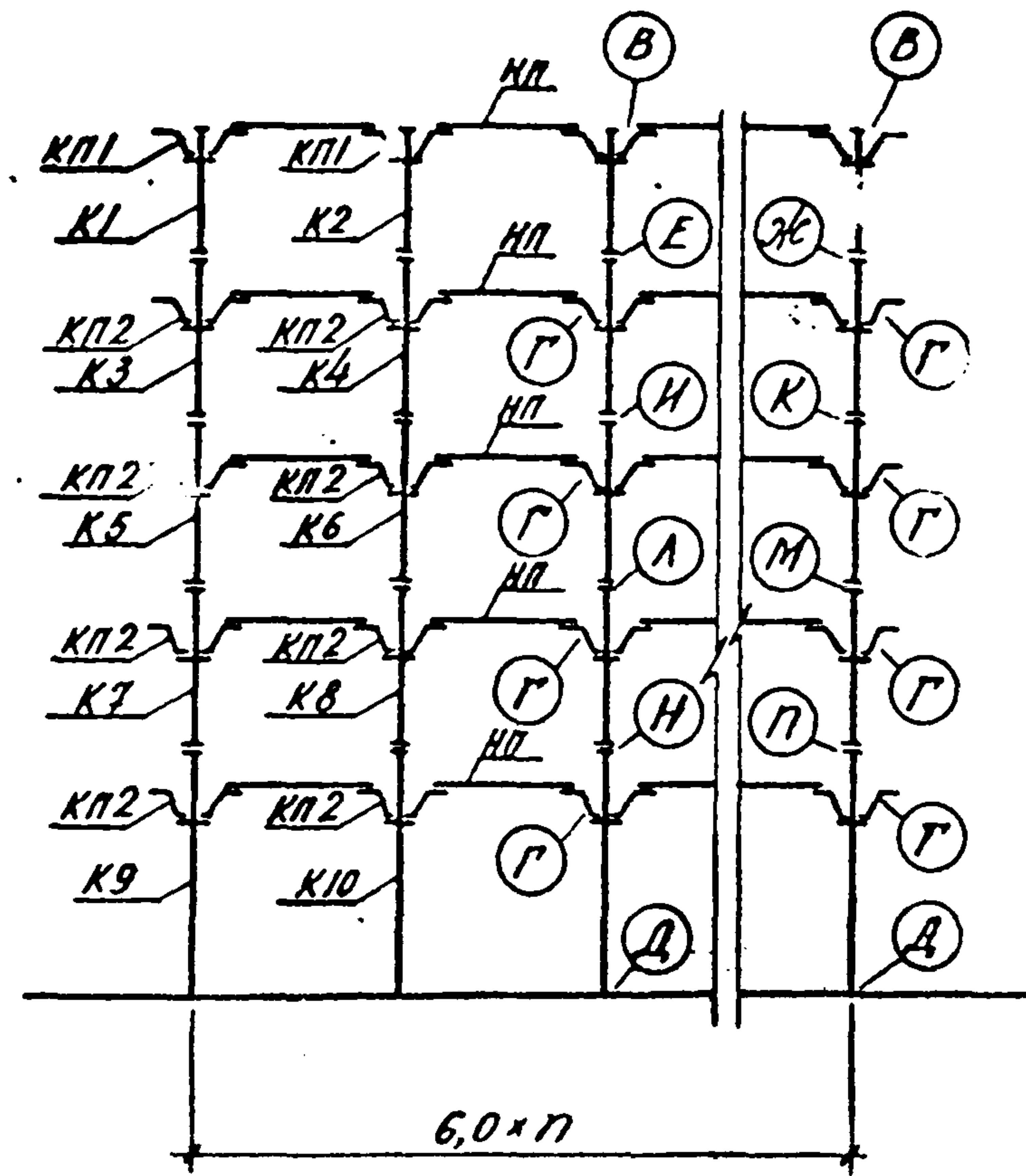
Схема рамы 6-1,55-π-5(4,8;4,8;6,0)
