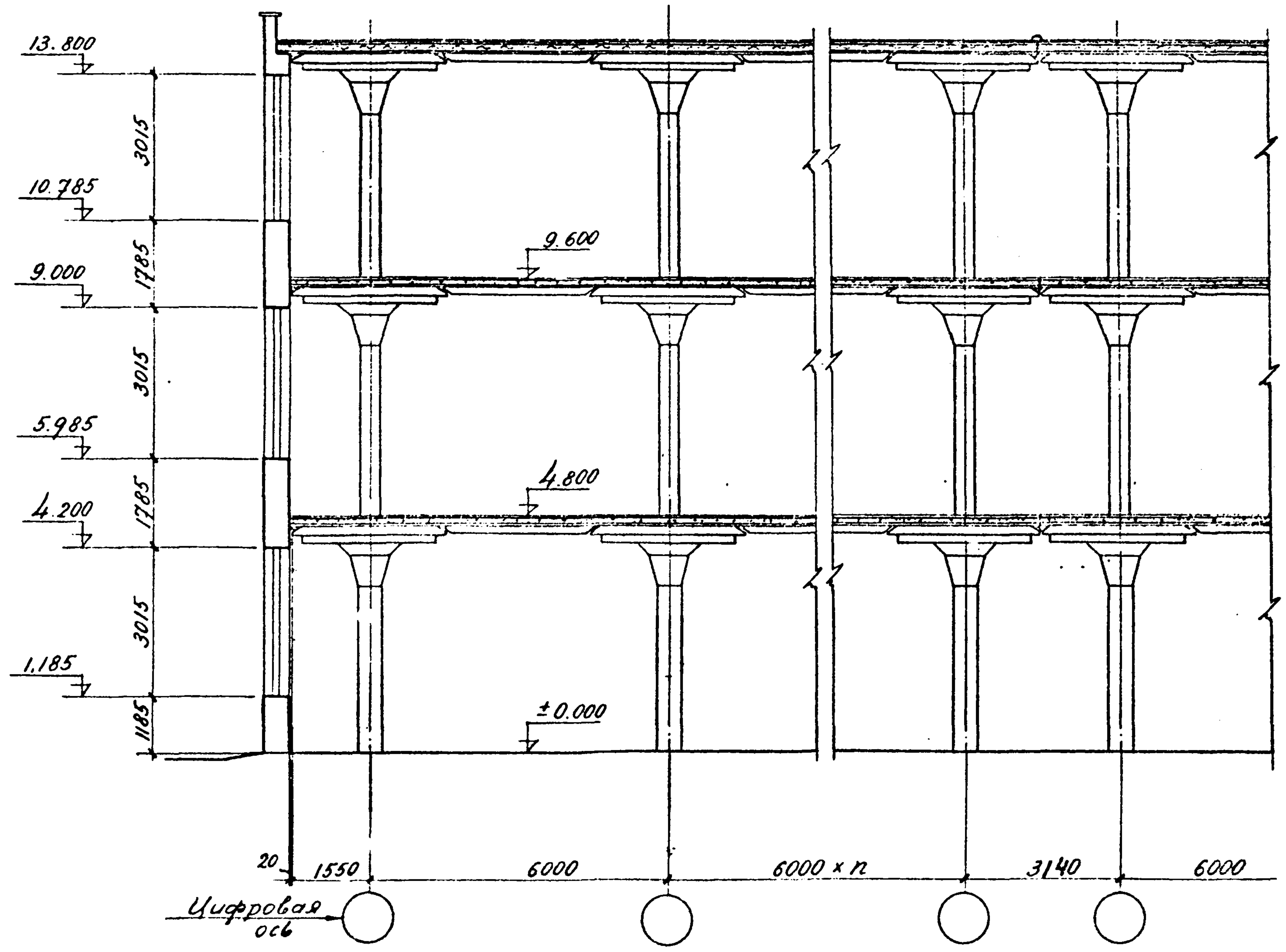
Продольный разрез (пример)
