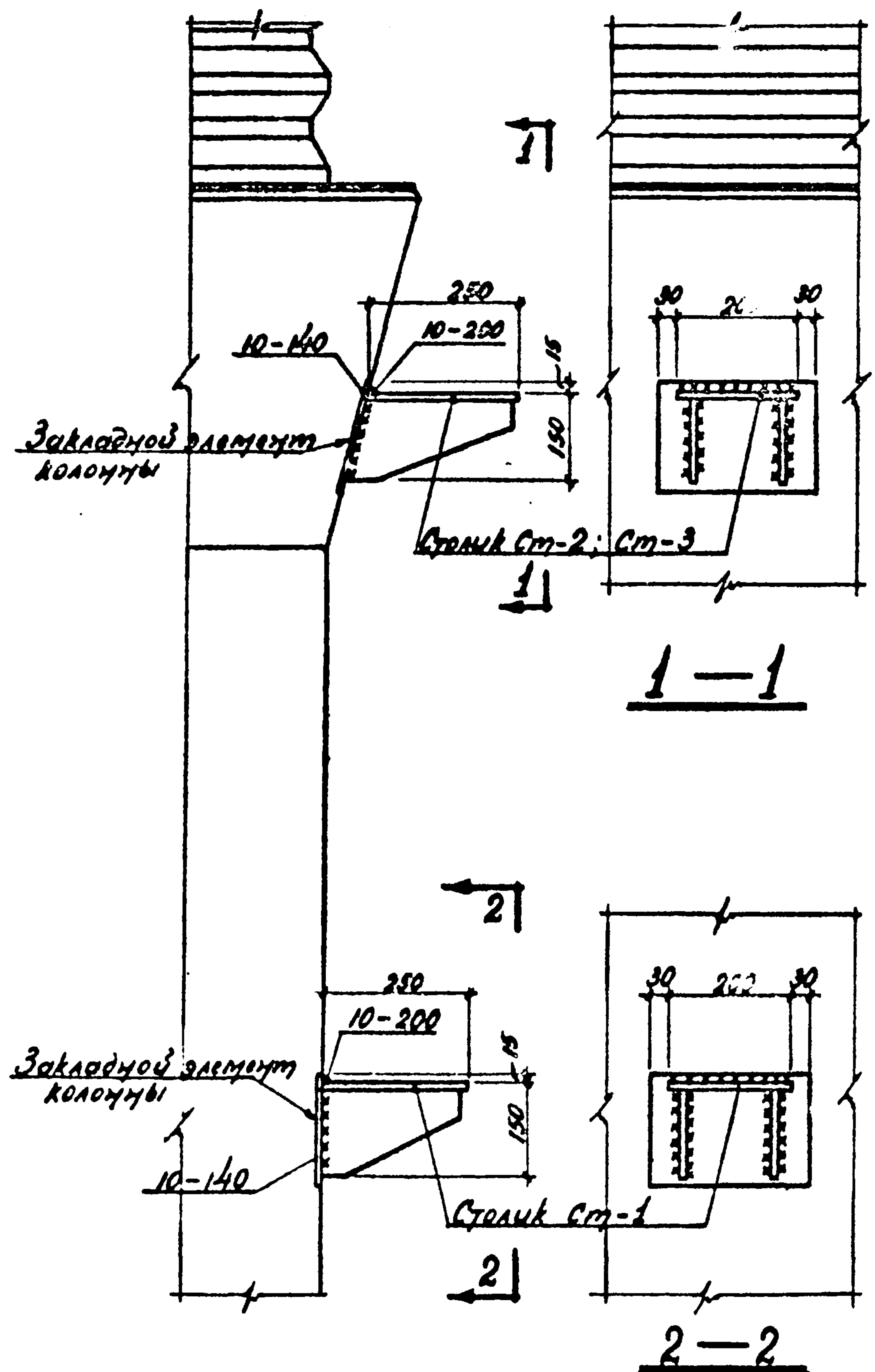
Примеры крепления столиков к закладным элементам колонн.
