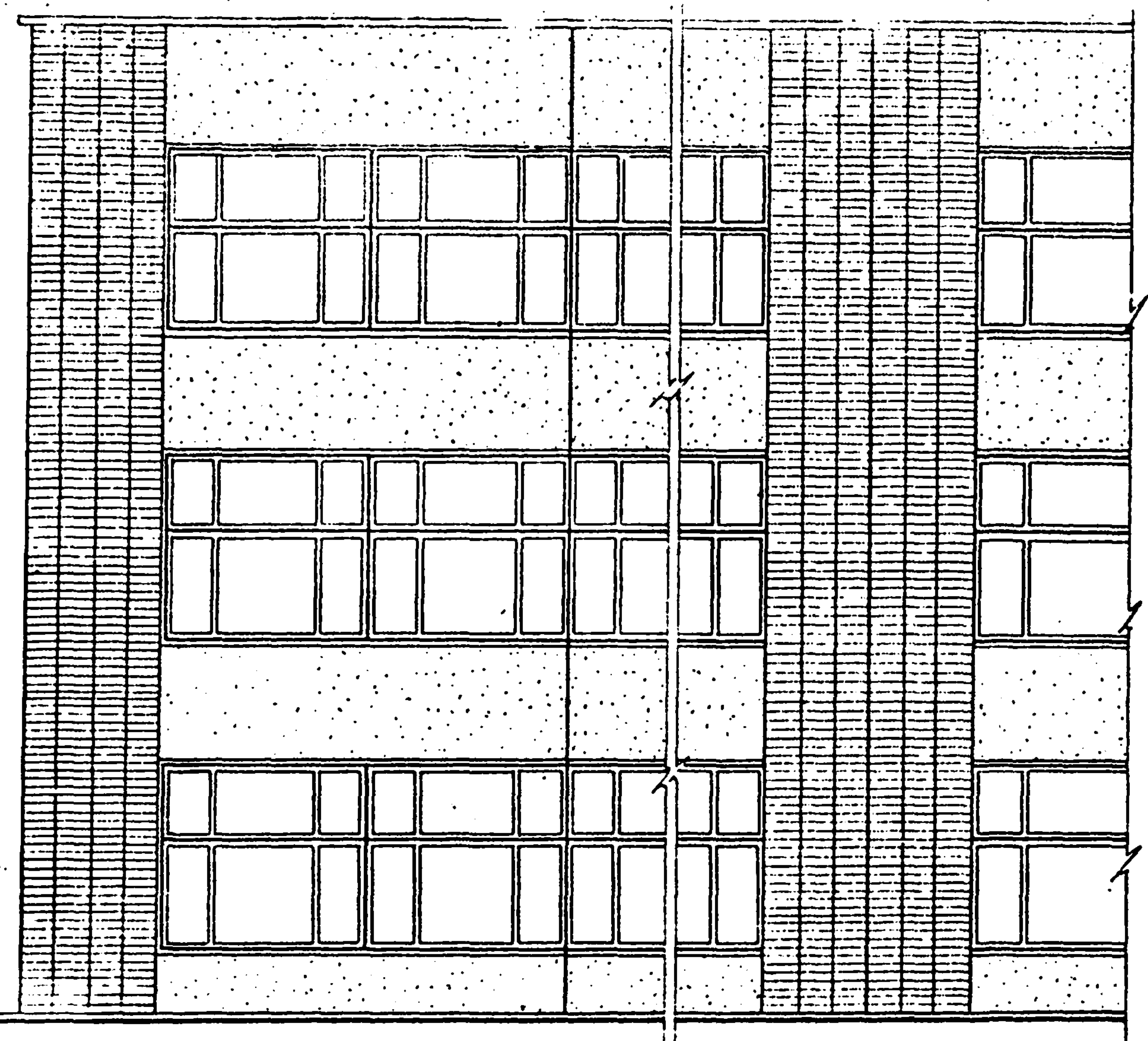
Фасад
