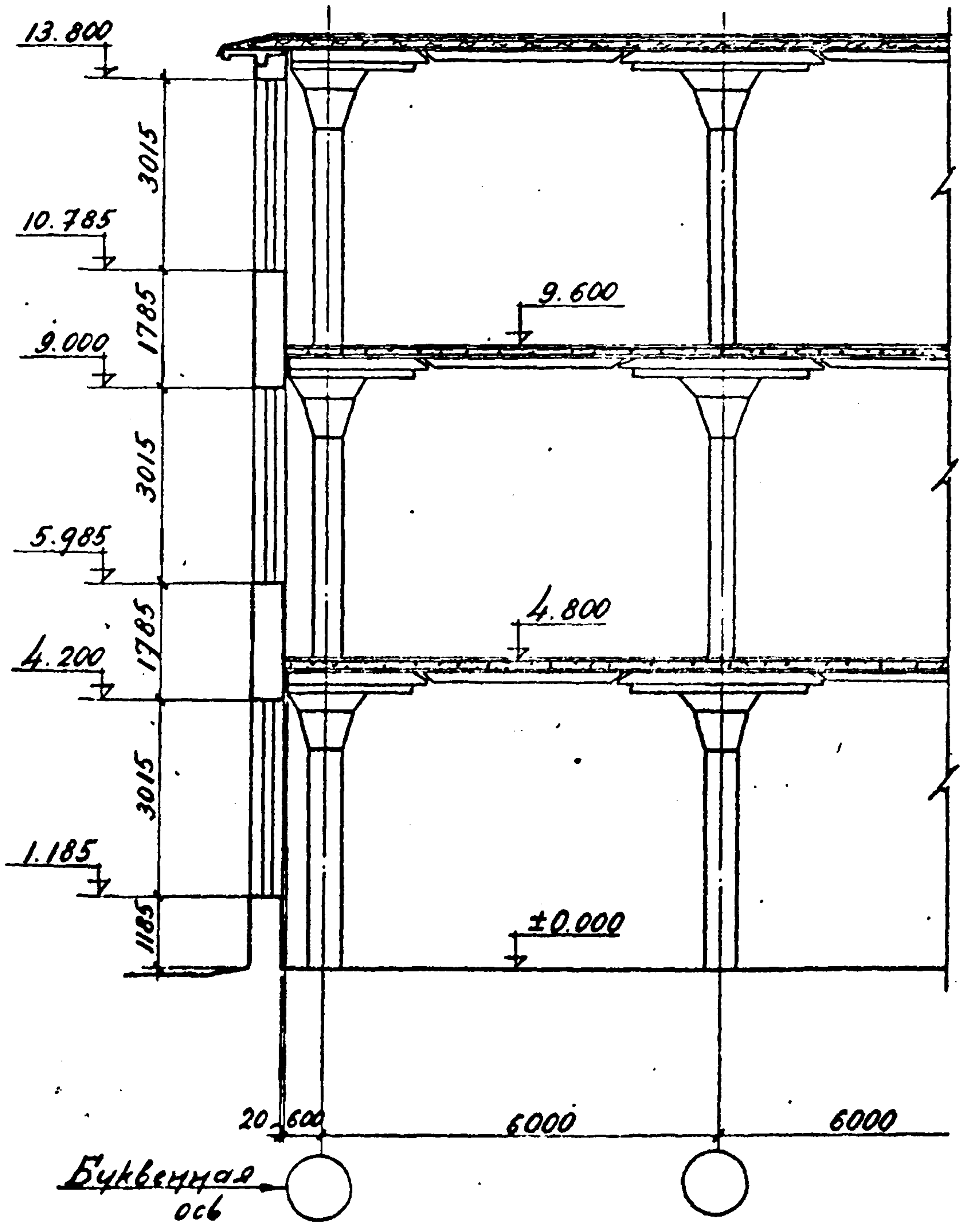
Поперечный разрез (пример)
