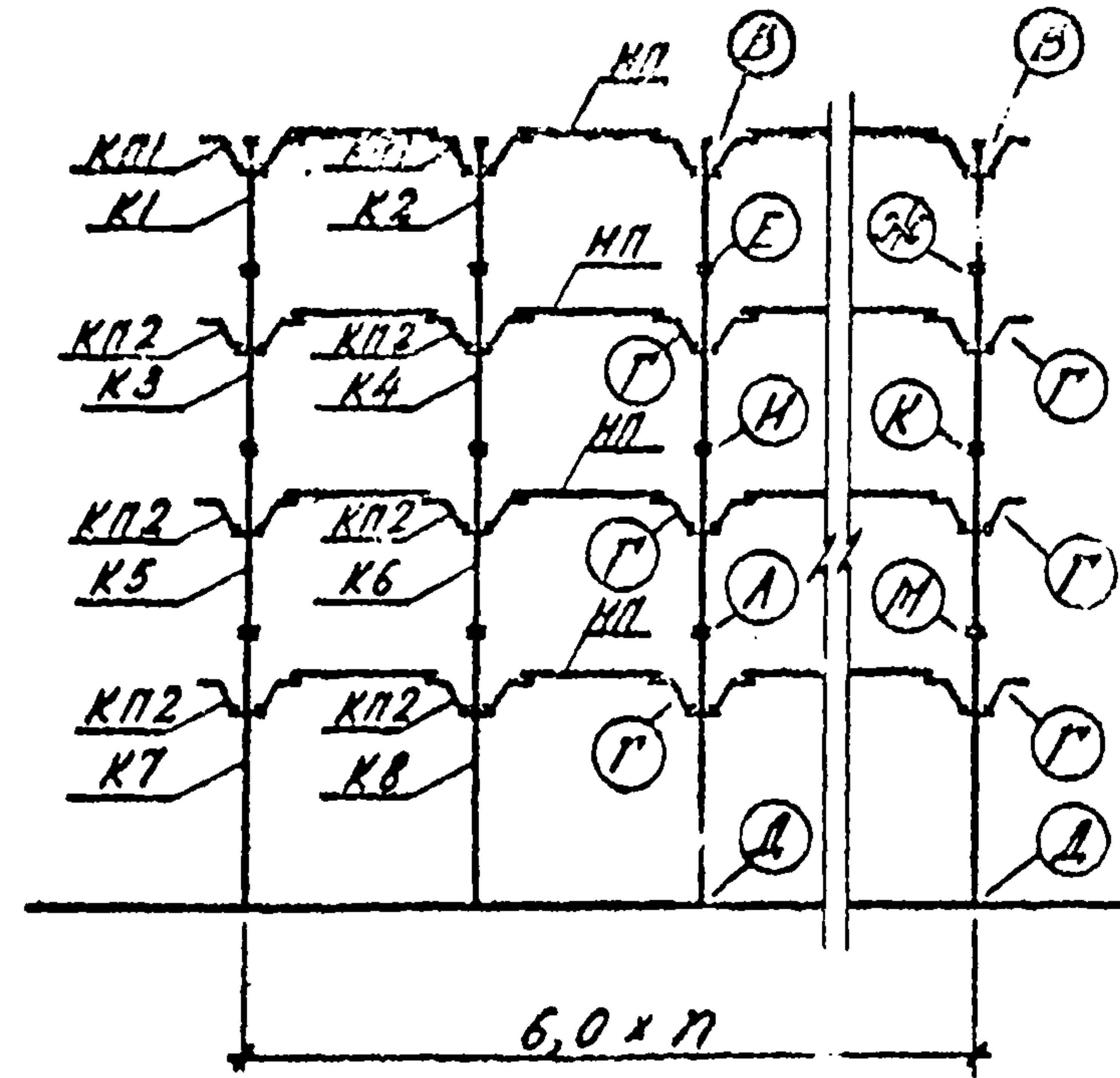
Схема рамы 6-1,55-п-4 (4,8; 4,8; 6,0)
