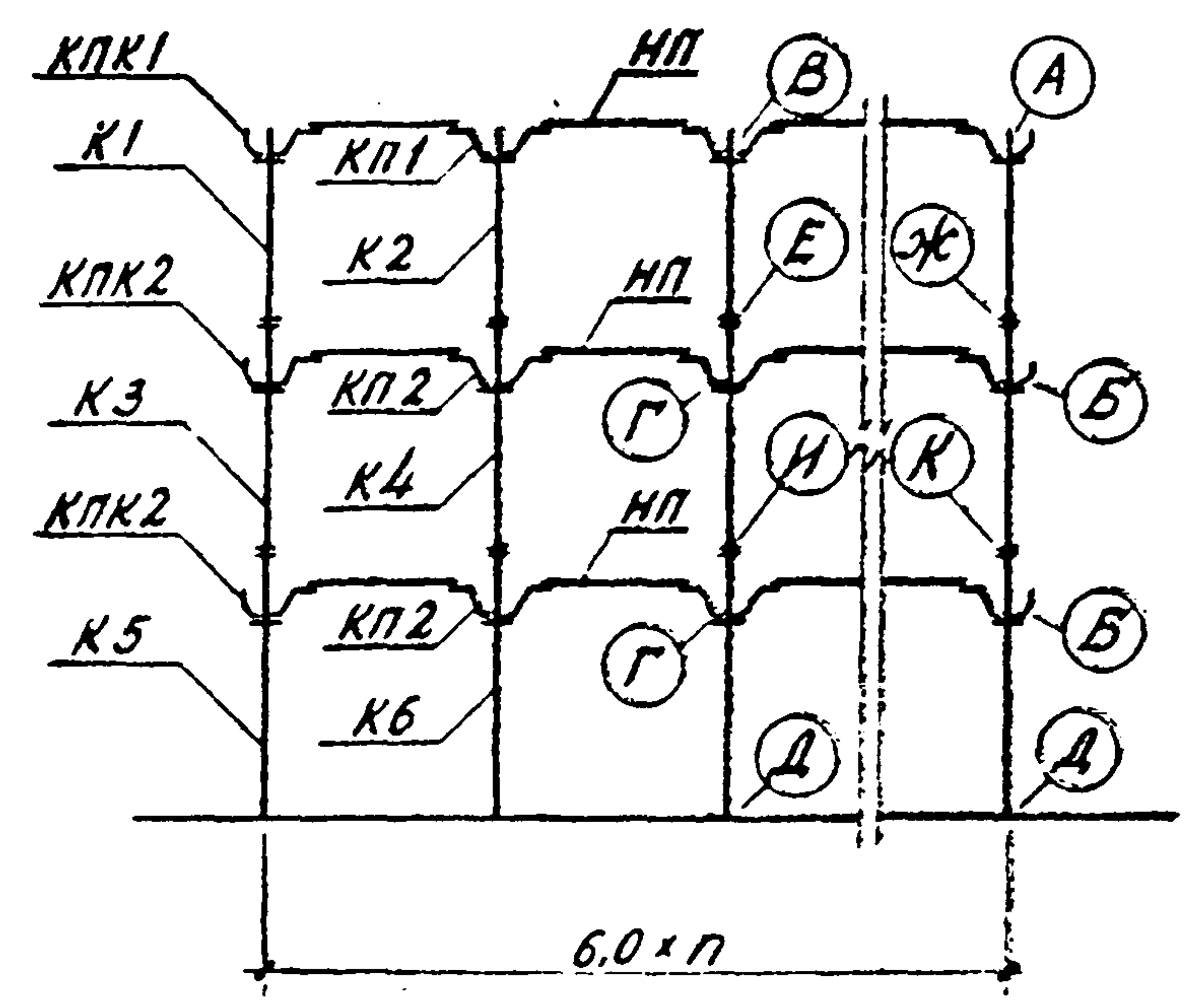
Схема рамы 6-0,6-п-3 (6,0)
