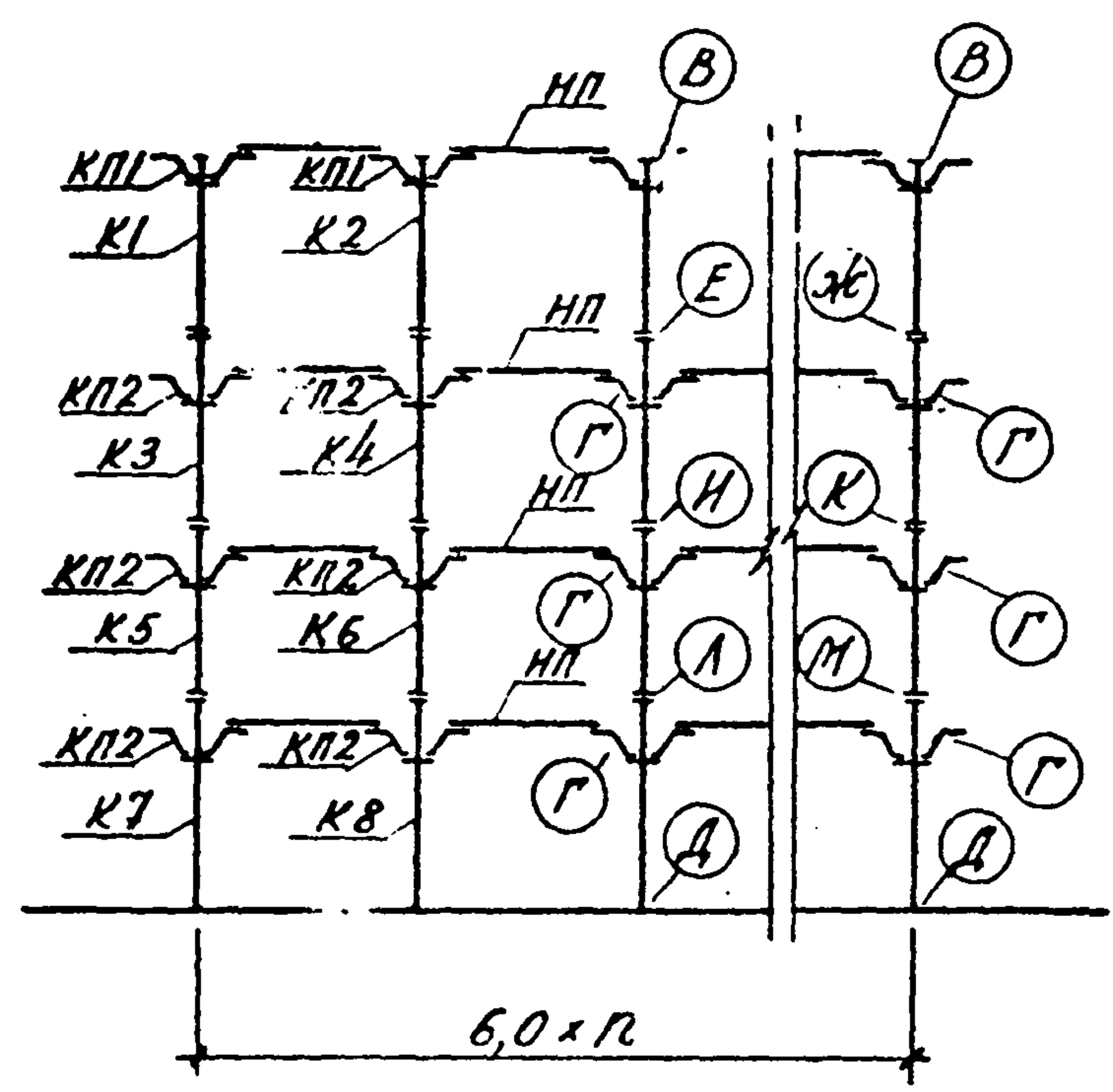
Схема рамы 6-1,55-12-4 (6,0; 4,8; 4,8)
