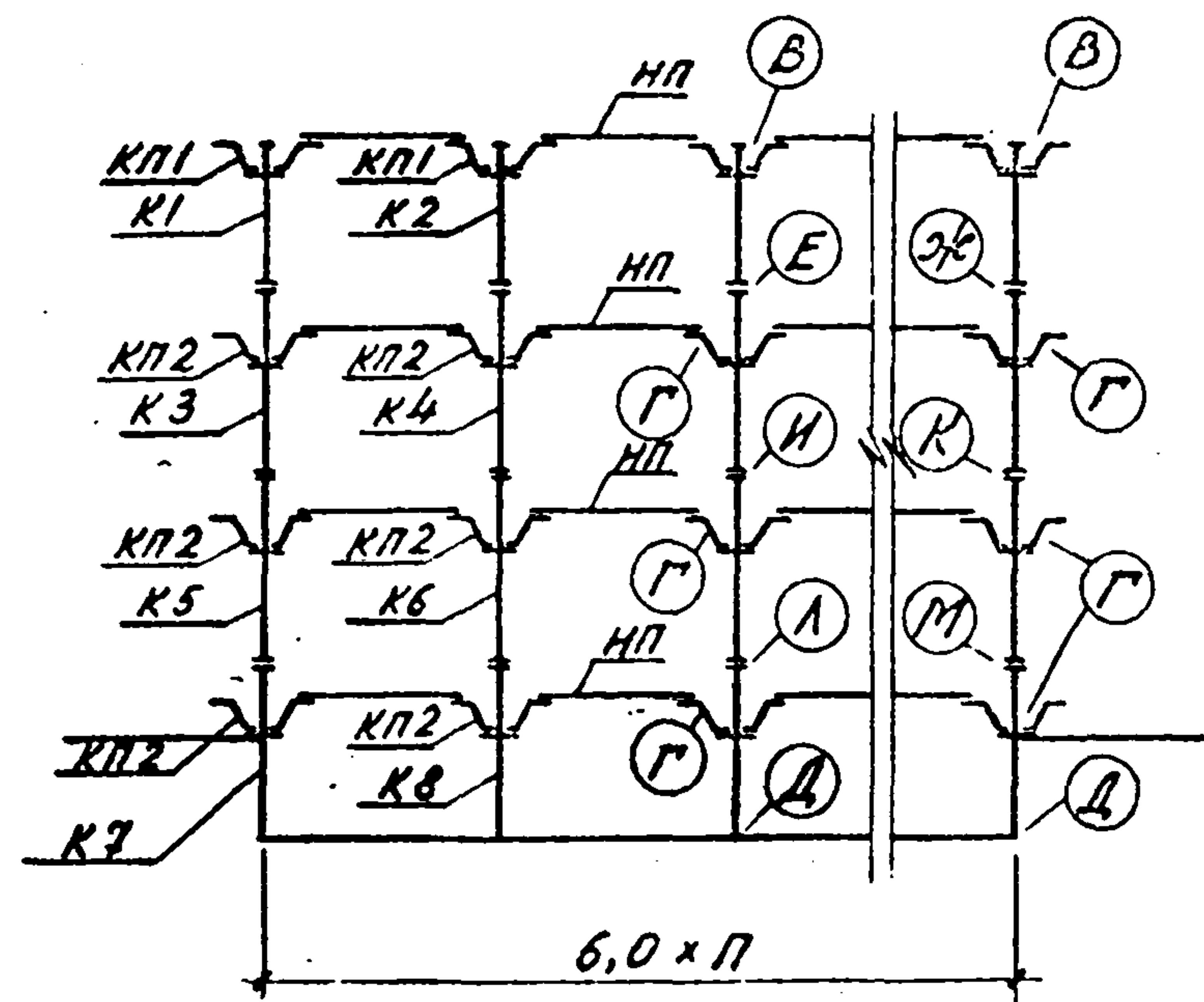
Схема рамы 6-1,55-п-3+подвал (4,8;4,8;3,6)
