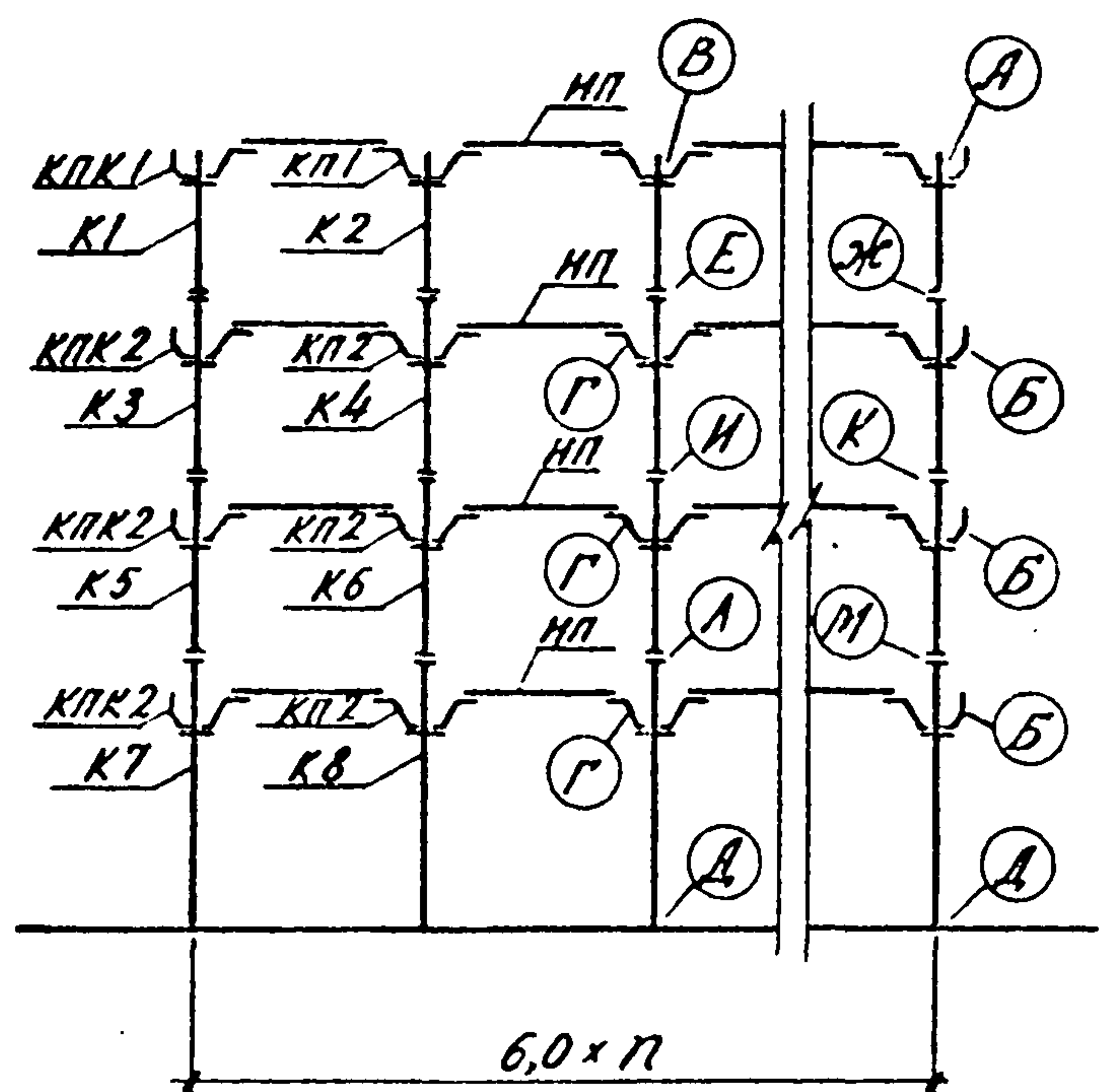
Схема рамы 6-0,6-n-4(4,8;4,8;6,0)
