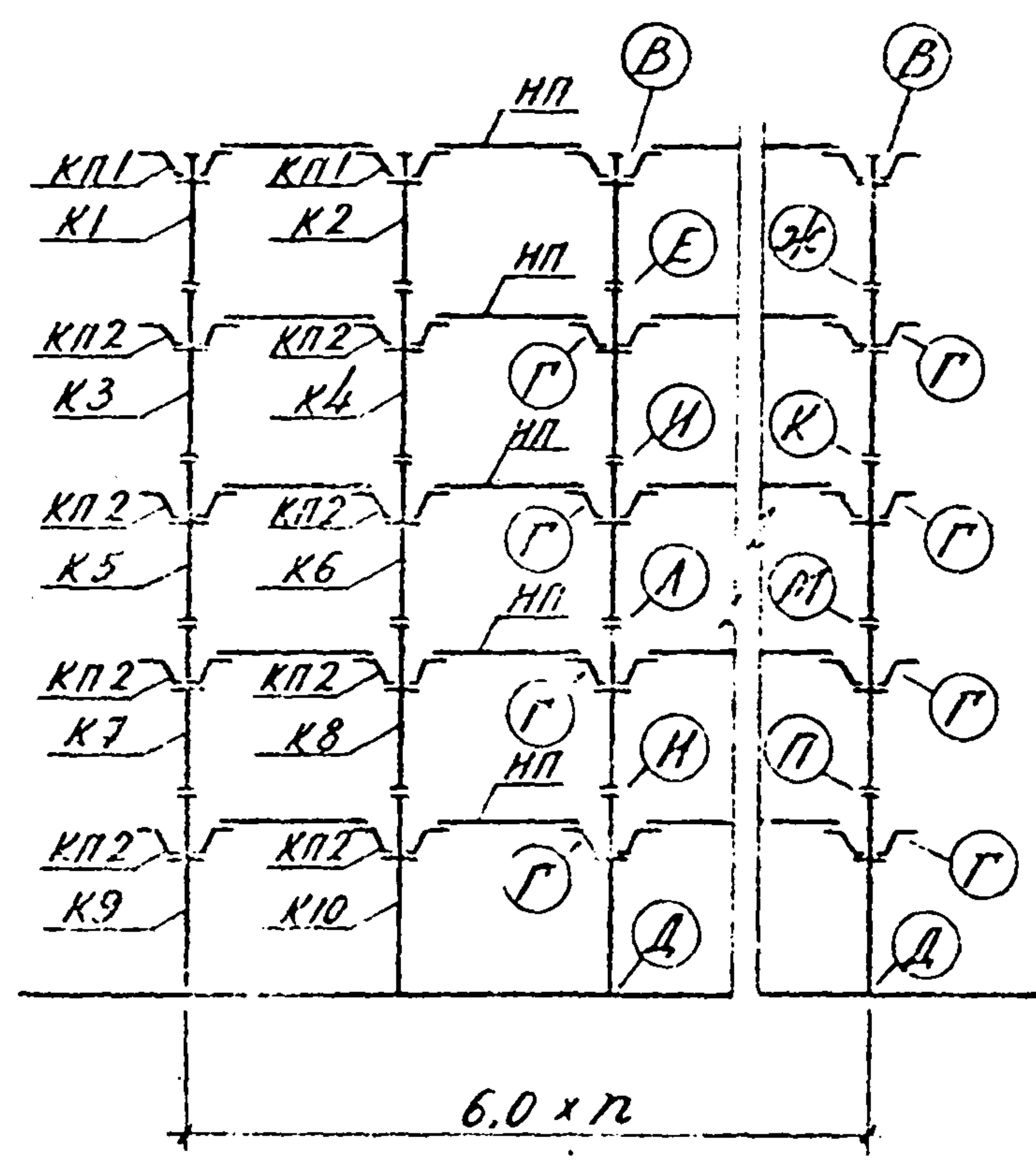
Схема рамы 6-1,55-П-5 (4,8)
