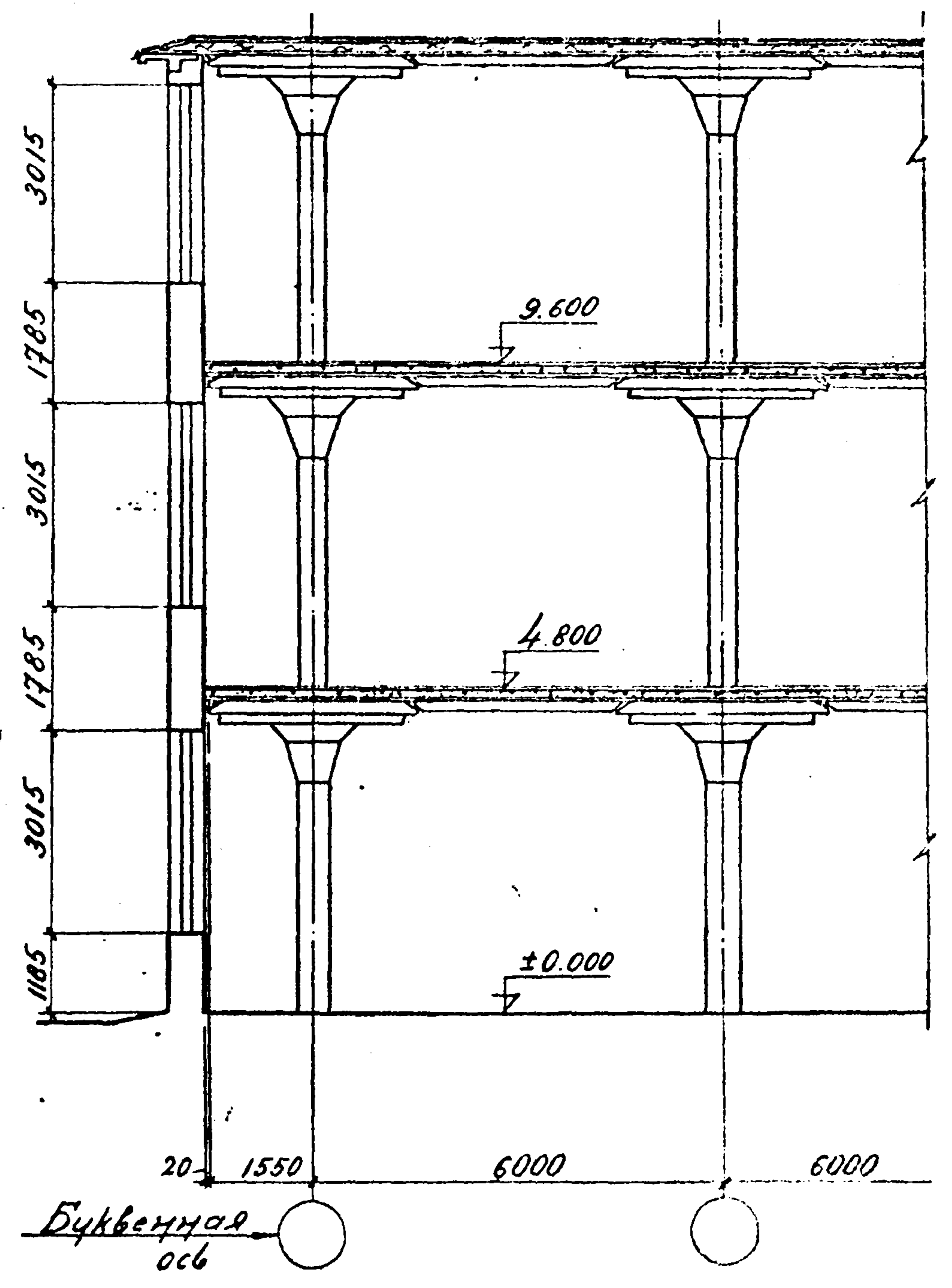
Поперечный разрез (пример)
