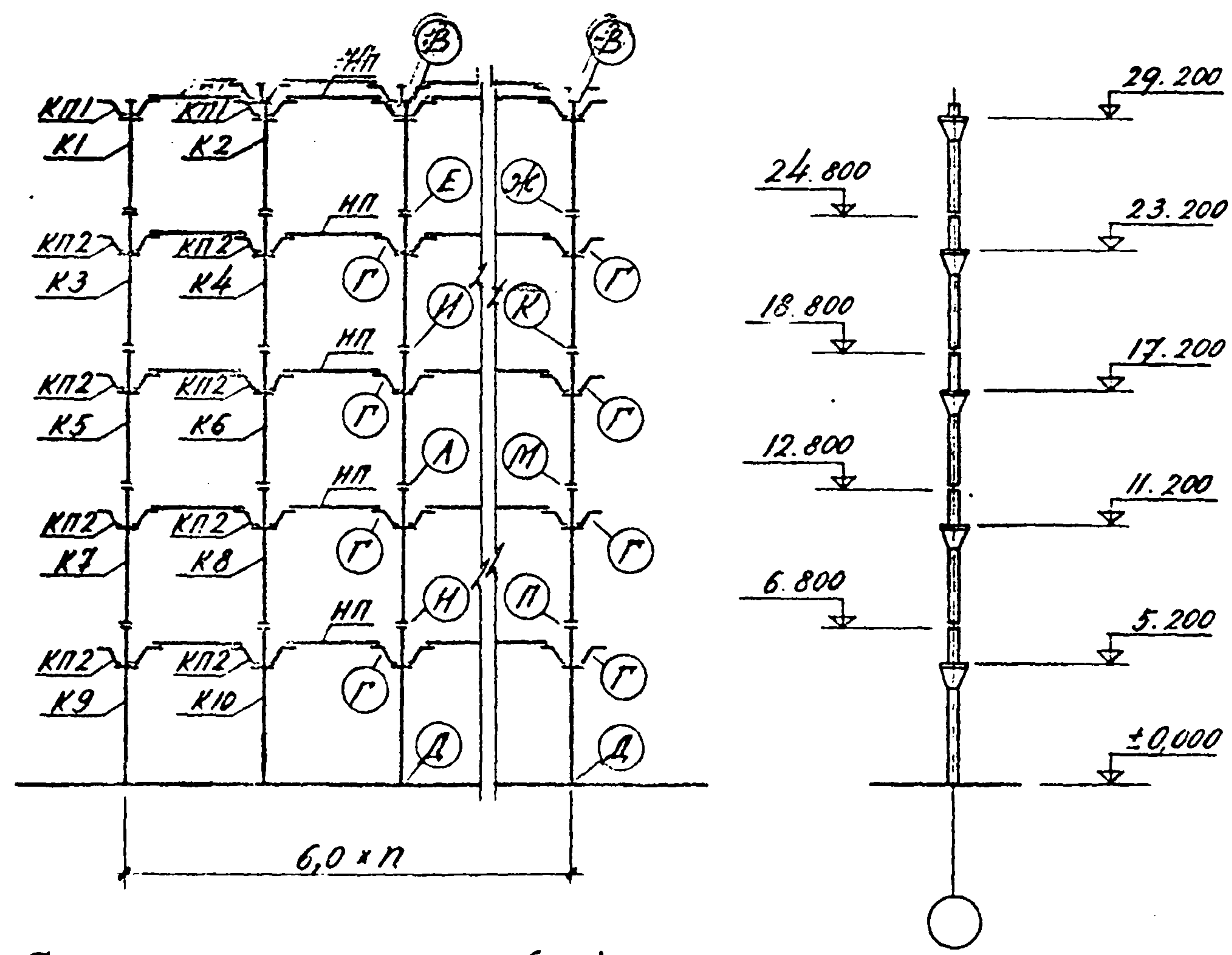
Схема рамы 6-1,55-п-5 (6,0)
