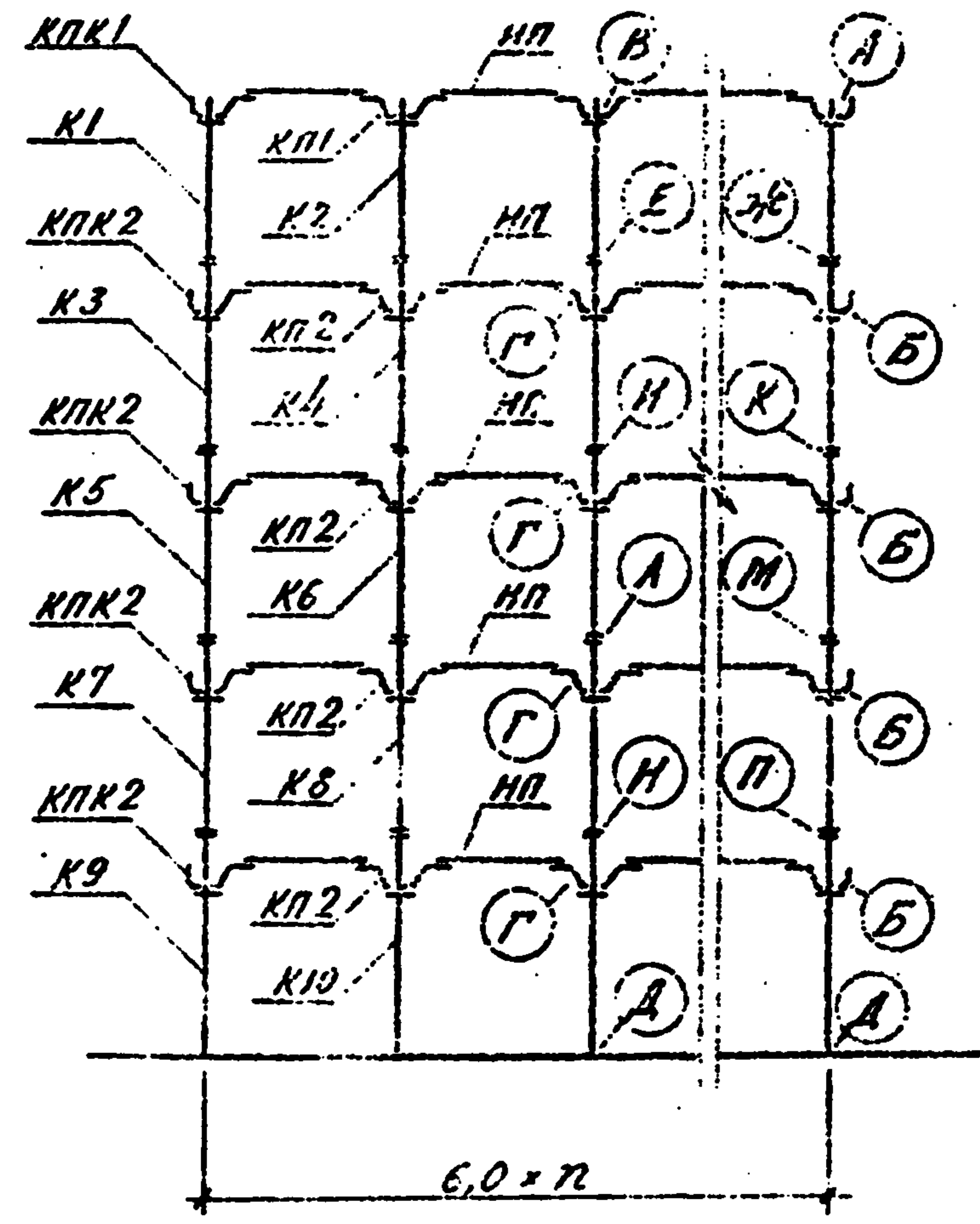
Схема рамы 6-0,6-п-5 (6,0)
