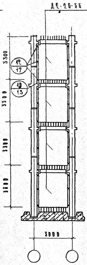
Диафрагмы в плоскости рам
