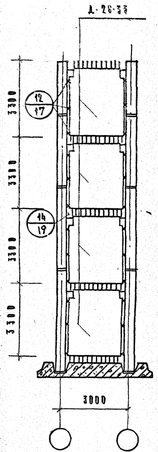
Диафрагмы перпендикулярные плоскости рам
