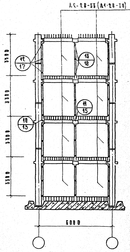
Диафрагмы в плоскости рам
