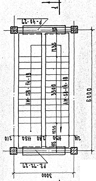
ЛЕСТНИЦА ДЛЯ ЭТАЖА С ВЫСОТОЙ ЭТАЖА 3.60М
