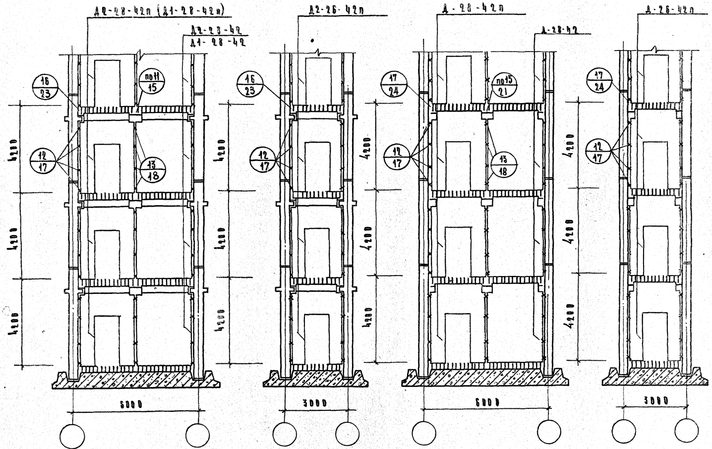
Диафрамы перпендикулярные плоскости рам
