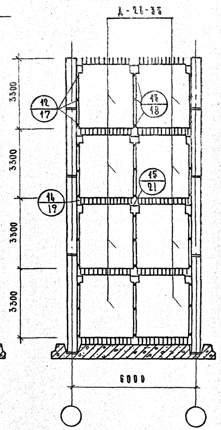
Диафрагмы перпендикулярные плоскости рам
